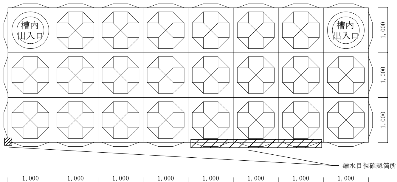
高置水槽平面図 S=1/50
