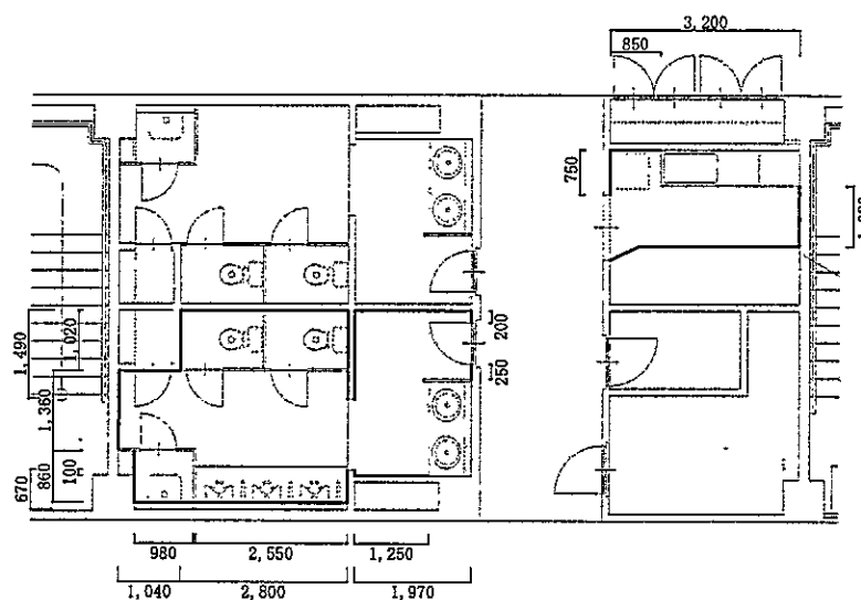
巾木撤去・新設平面図
