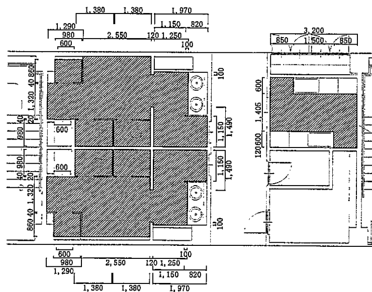
床撤去・新設平面図
