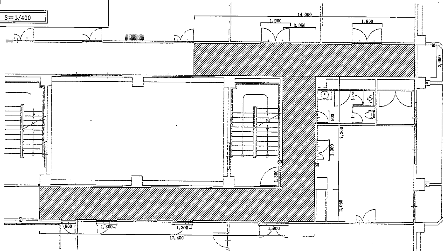
291号建物2F（撤去・新設）平面図 S=1/100
