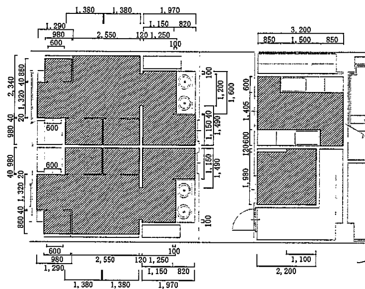
床撤去・新設平面図
