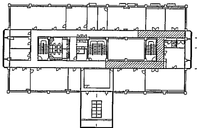
290号建物2F平面図 S=1/400
