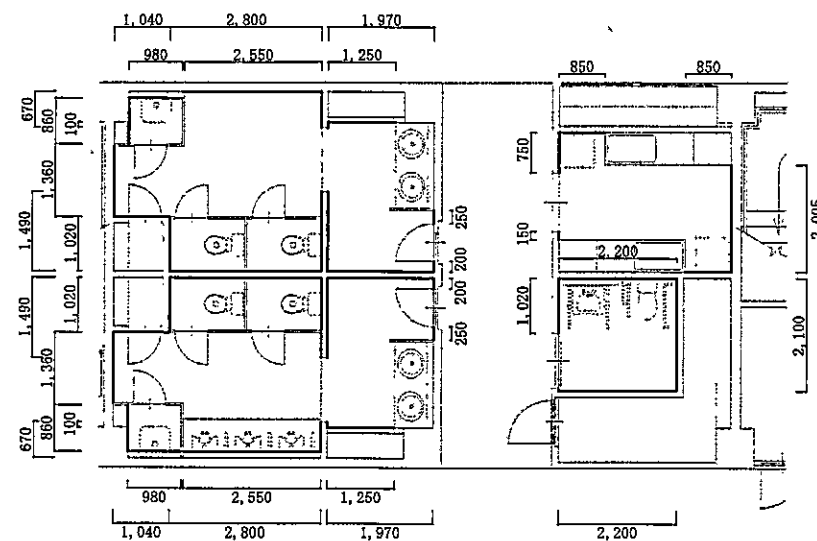
巾木撤去・新設平面図
