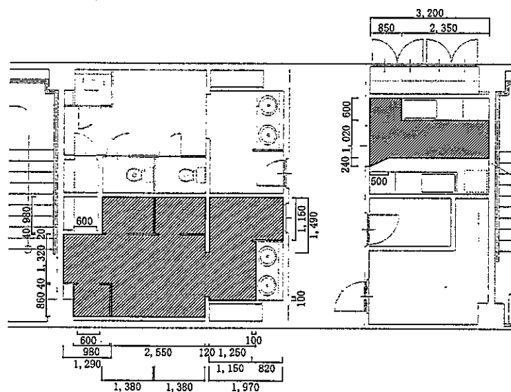
床撤去・新設平面図
