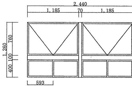
網戸新設予定窓枠A S=1:50
