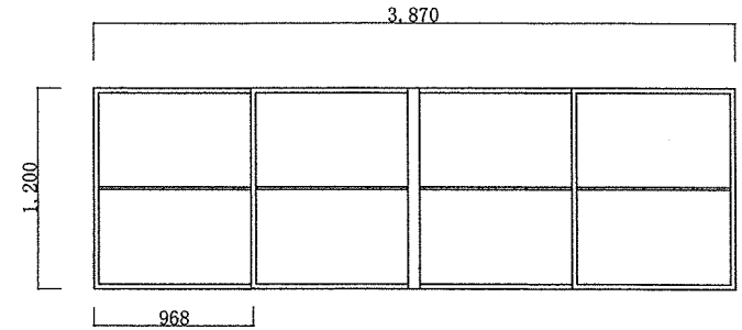
網戸新設予定窓枠D S=1:50
