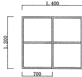
網戸新設予定窓枠B S=1:50
