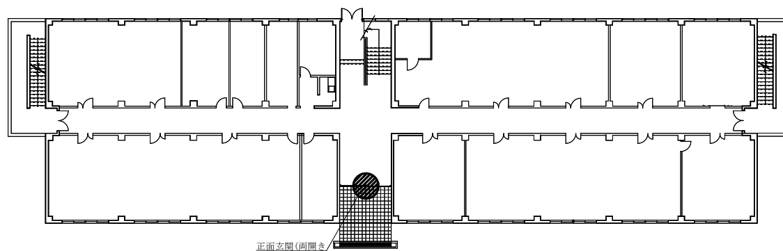
116号建物平面図 S=1/300
