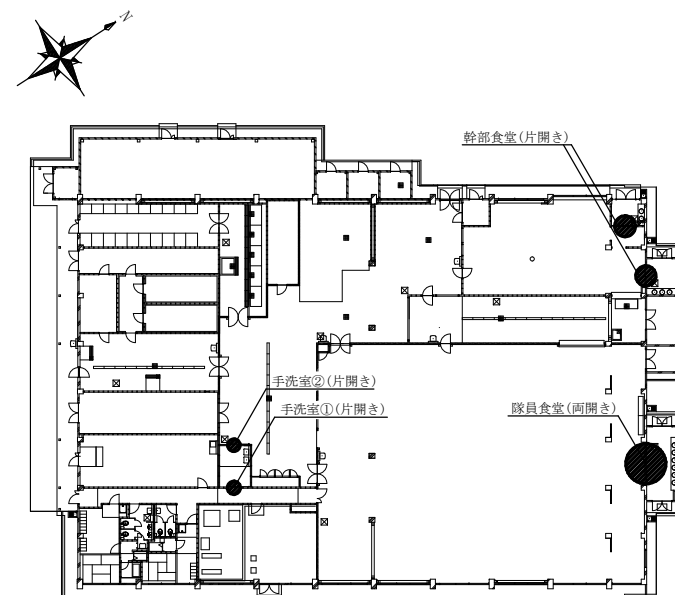
112号建物平面図 S=1/500
