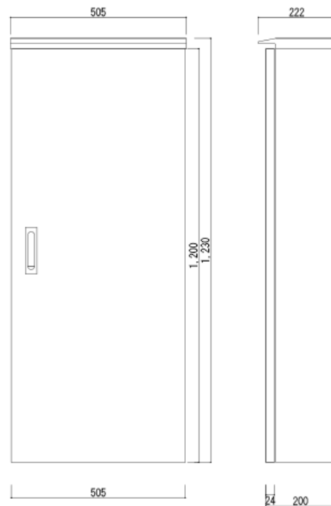
動力分電盤
