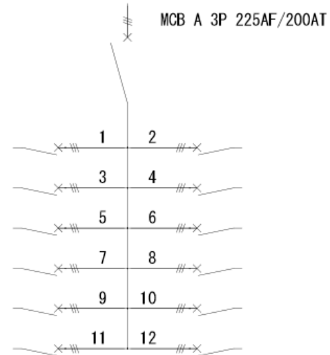
1～12 : MCB 3P 50AF/30AT 各1個
