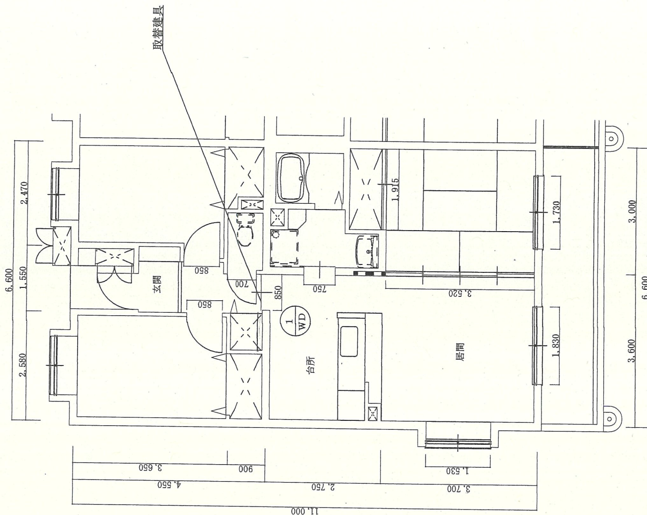
大豆田 平面図 (基準) S=1/80
