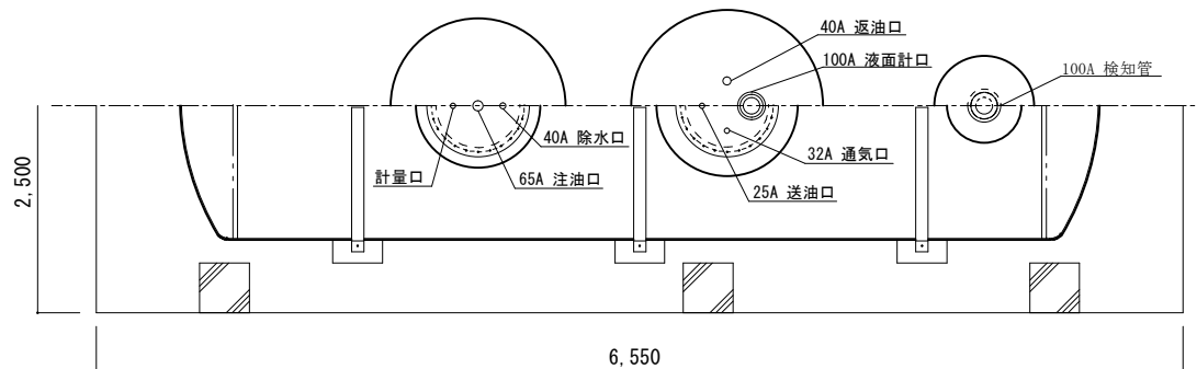
燃料地下タンク平面図 1 / 5 0
