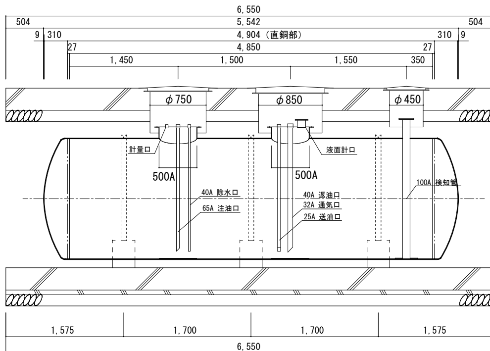
燃料地下タンク断面図 1 / 5 0
