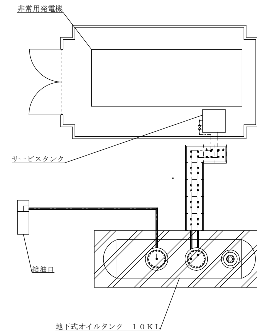
非常用発電機室平面図 1 / X
