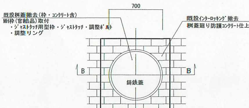
汚水平マンホール平面図 S=1:30
