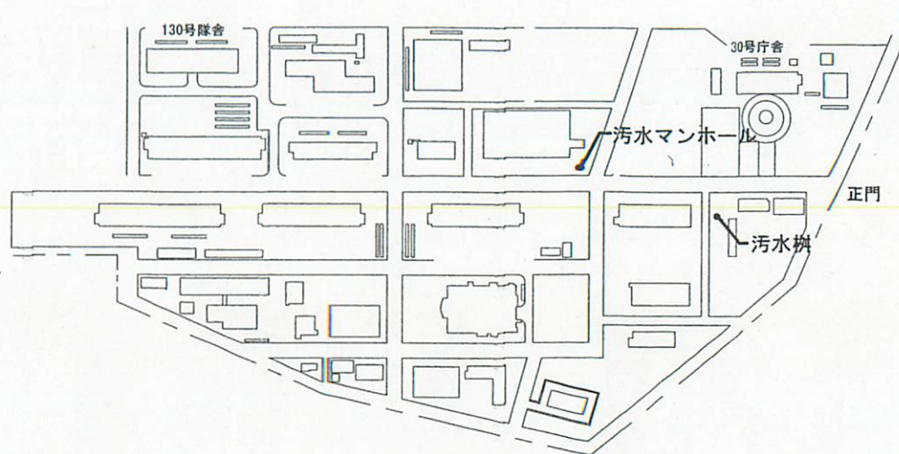
配置図 S=1/5000
