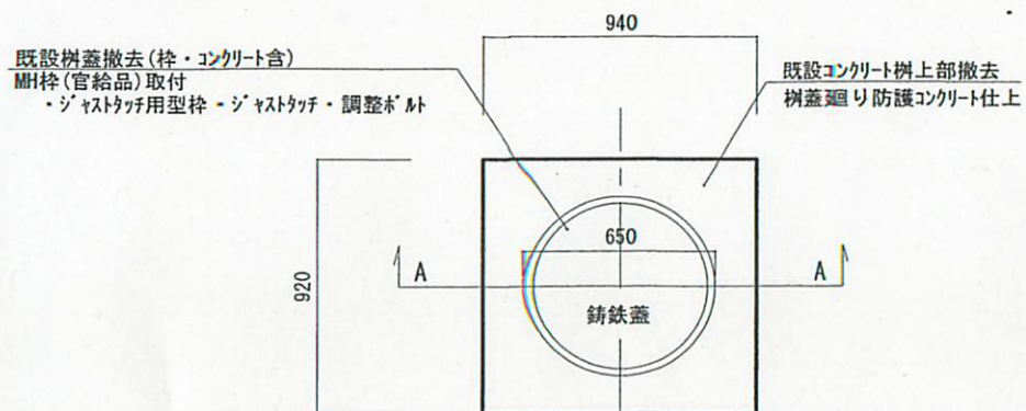
汚水枘平面図 S=1:30
