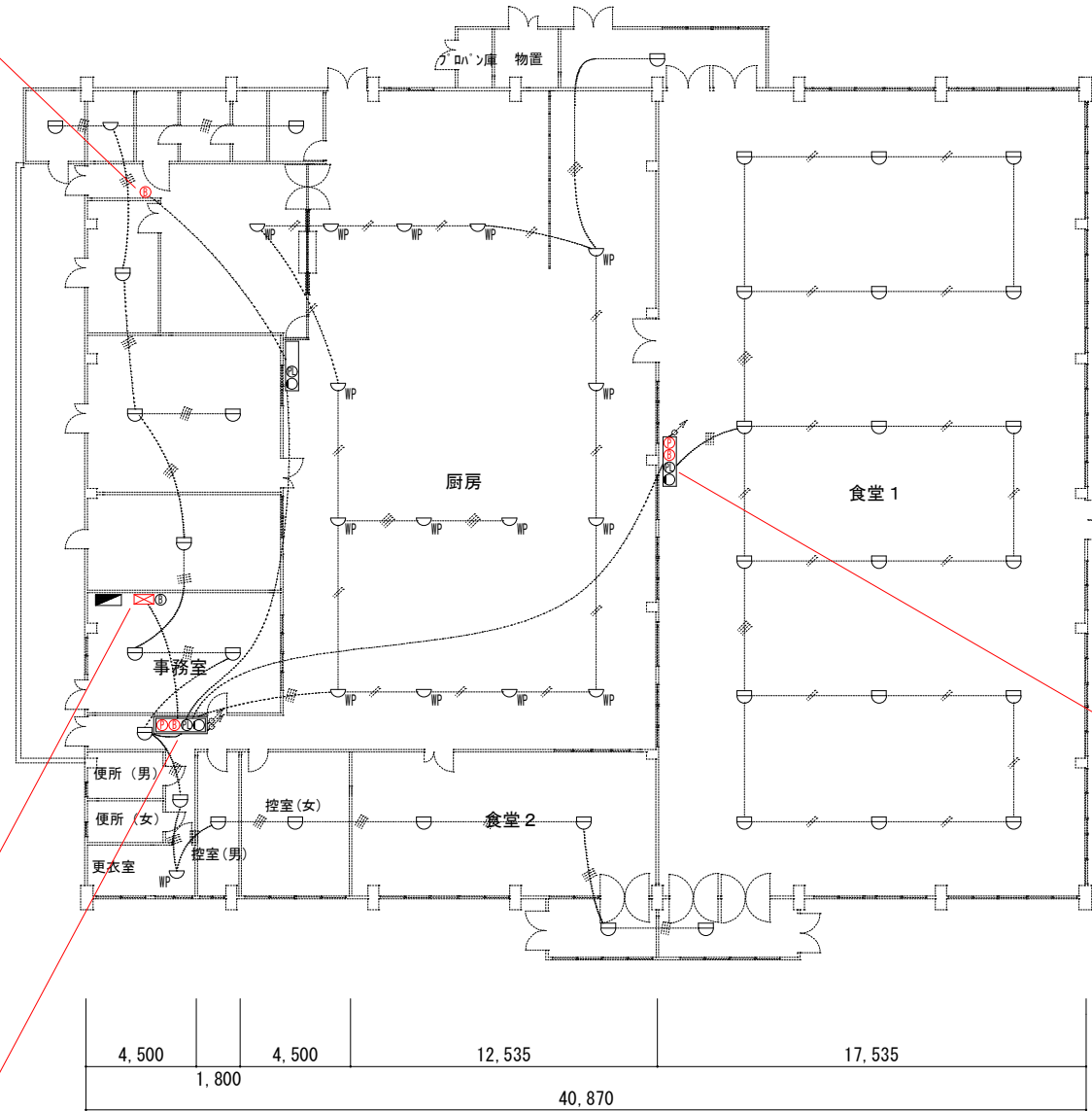
自動火災報知設備配置図（1階） S=1/300
