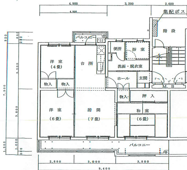
作業場所 平面図 S=1/100
