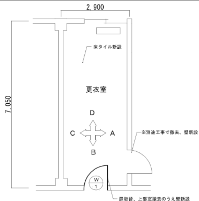
改修後 1階更衣室平面図 S=1/100
