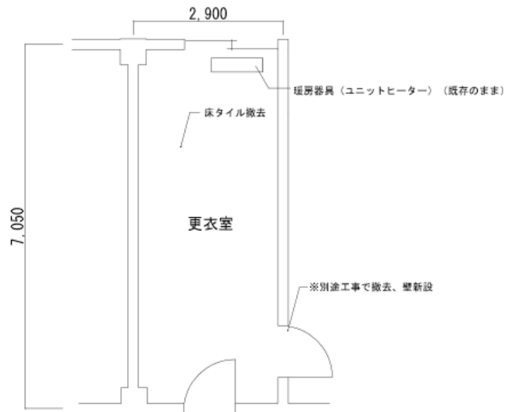
改修前 1階更衣室平面図 S=1/100
