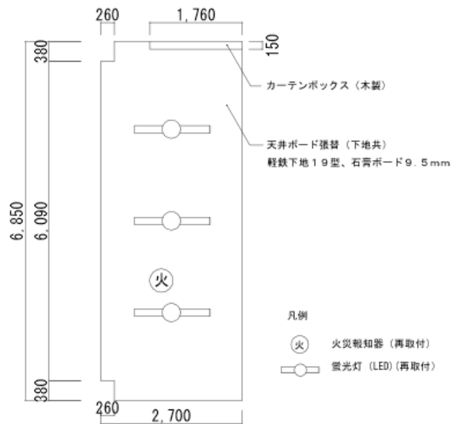
改修後 1階更衣室天井伏図 S=1/100
