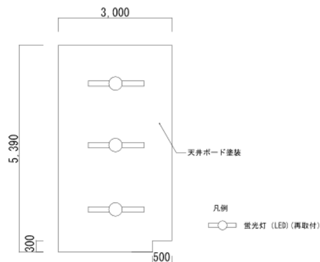
改修後 1階更衣室2天井伏図 S=1/100
