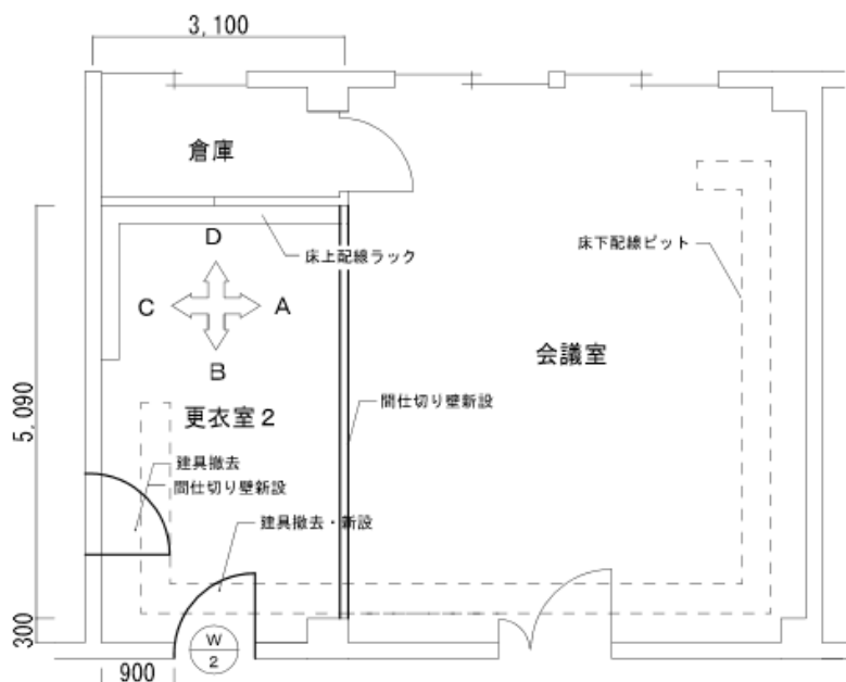
改修後 1階会議室平面図 S=1/100
