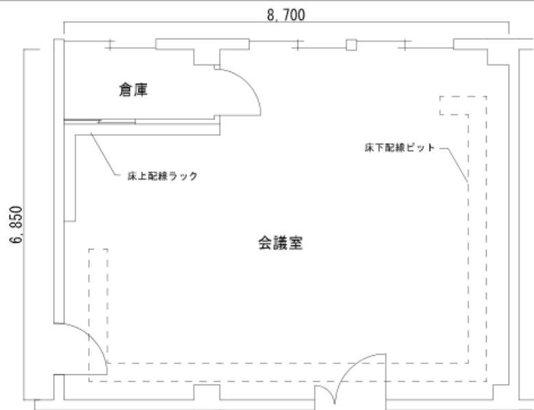
改修前 1階会議室平面図 S=1/100
