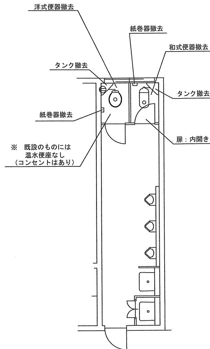
現況図 1:100
