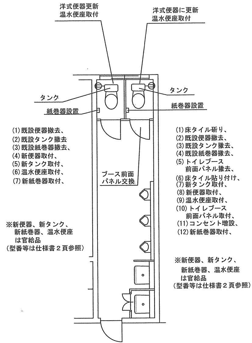
改修図 1:100
