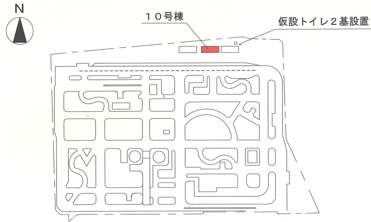
自動車訓練場配置図 S=1/1,500
