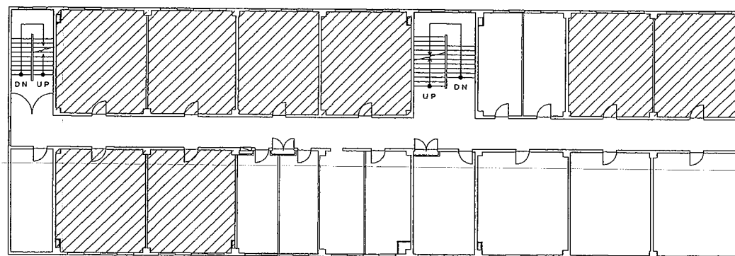
77号建物2階平面図
