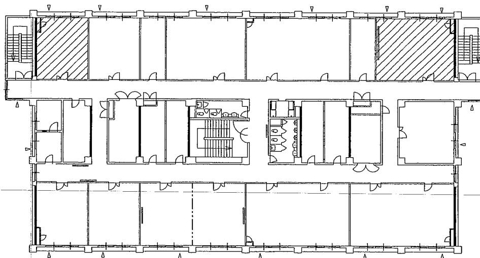
140号建物4階平面図
