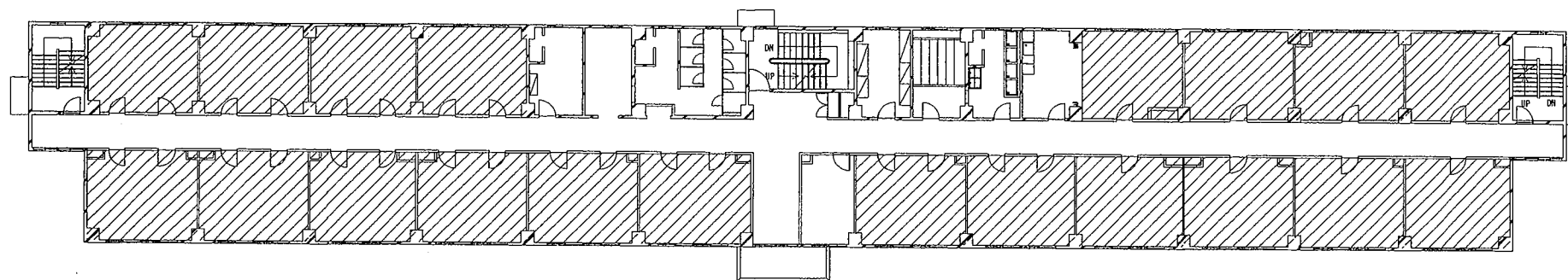
117号建物2階平面図
