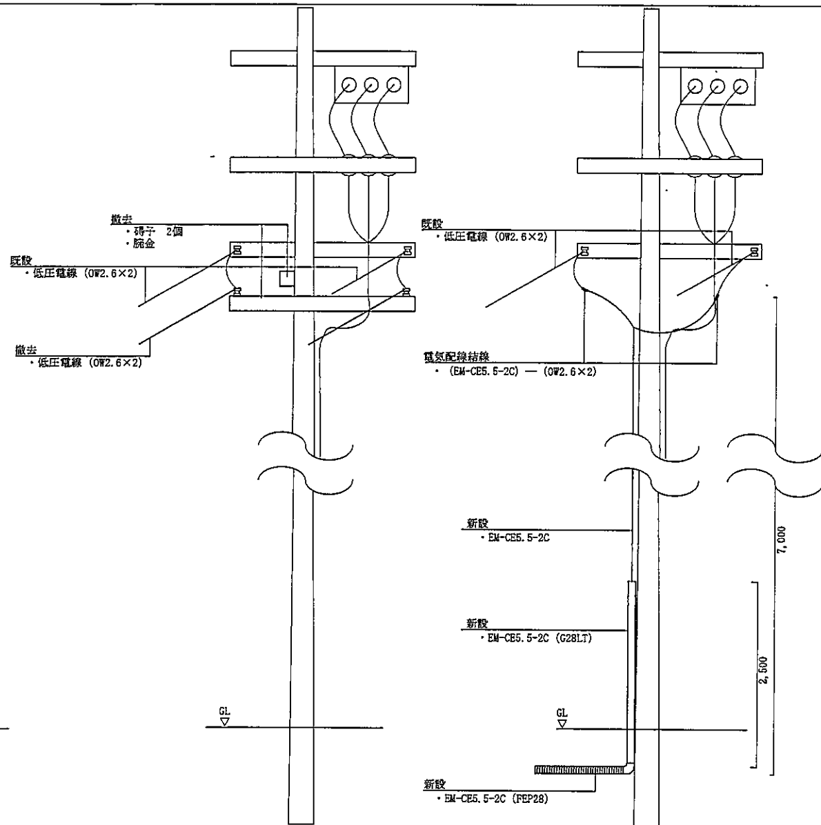
装柱撤去図
