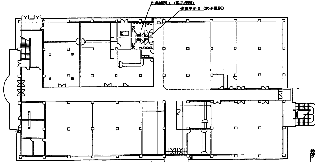
115号建物1階平面図 S = 1 / 5 0 0
