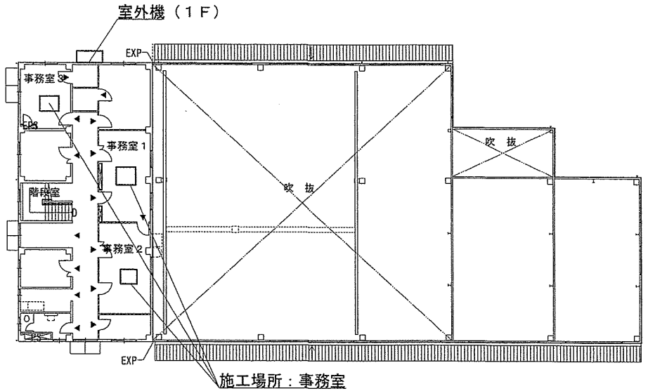
整備工場2階平面図・詳細図 S=1:400
