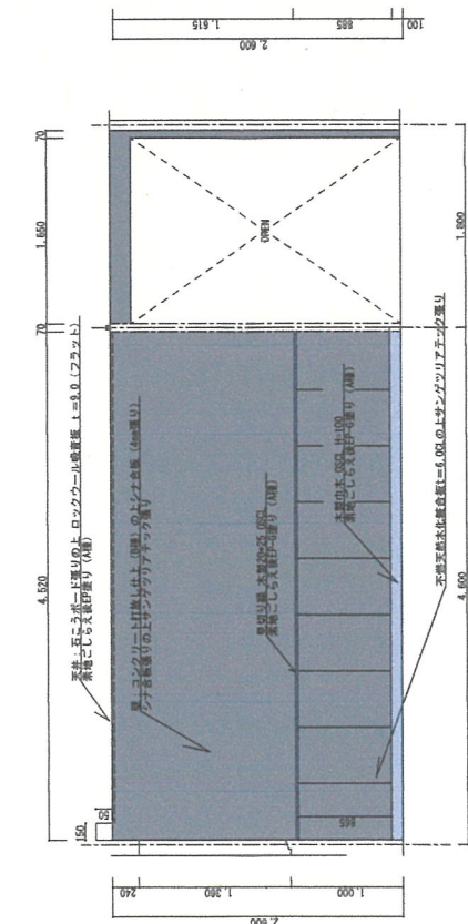
A面展開図 (改修後) S=1/50
