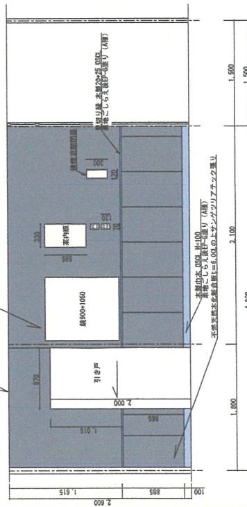
G面展開図 (改修後) S=1/50
