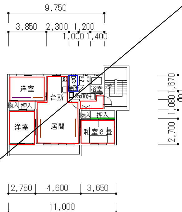
9号室平面詳細図（基準階）
