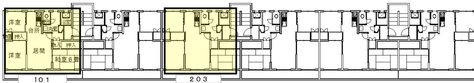
新川宿舎平面図（基準階）
