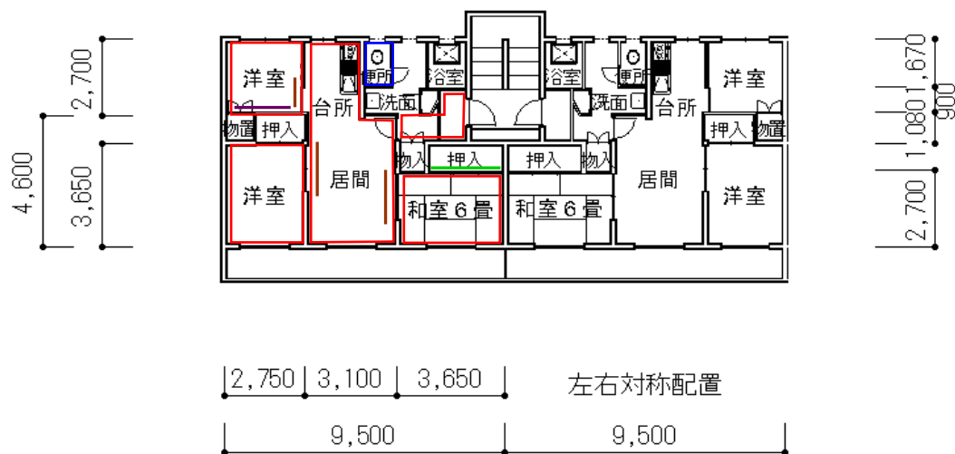
1～6号室平面詳細図（基準階）
