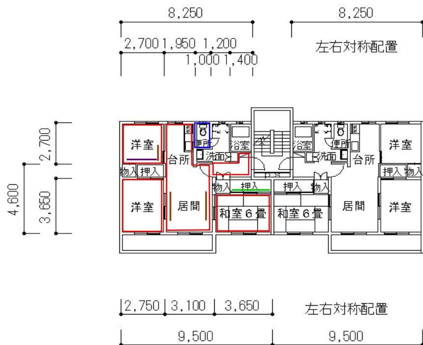
1～8号室平面詳細図（基準階）
