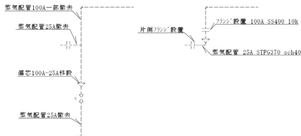
配管補修前詳細図 1 : 10
