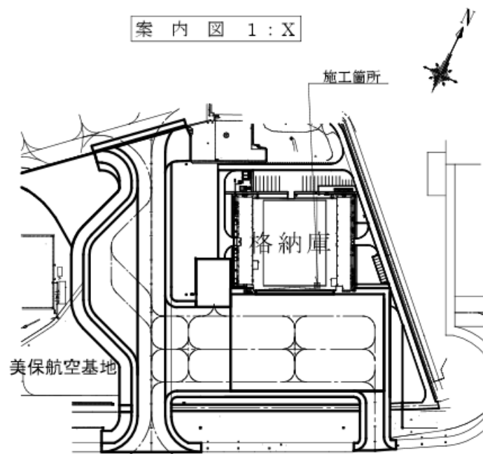
分屯地配置図 1 : X
