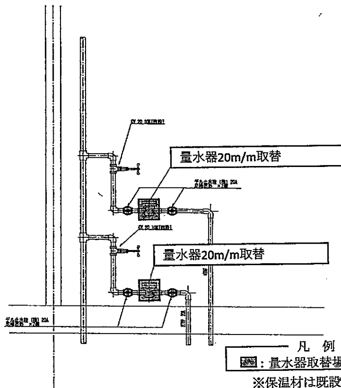
MB内取替図 (標準)
