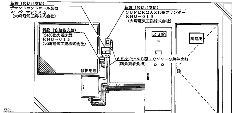
事務室B面立面図 (作業後) S=1/30
