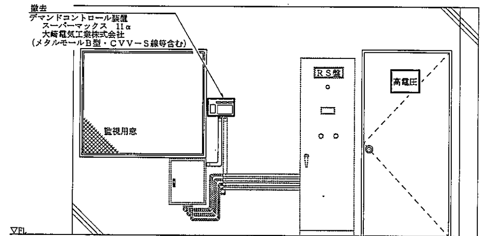
事務室B面立面図 (作業前) S=1/30
