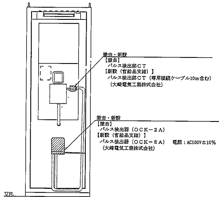
高压受電設備機器A面立面図 (作業前・後) S=1/20
