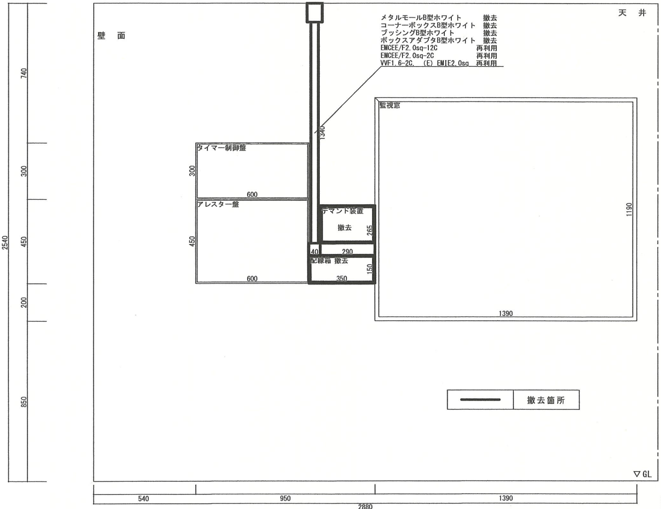
立面（撤去）
