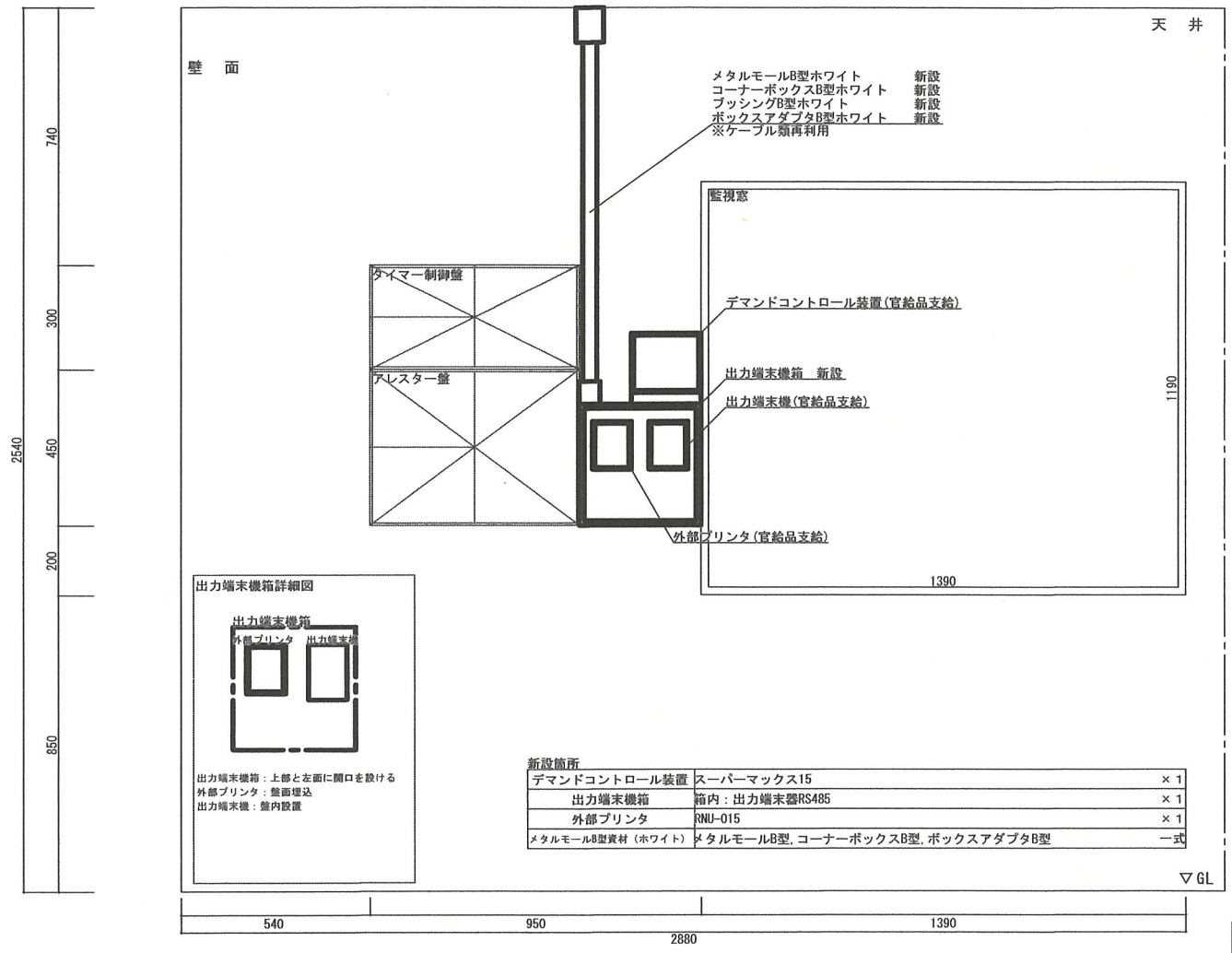
立面（新設）
