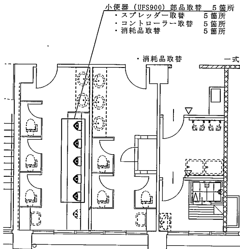
300号建物 (2F 男子トイレ) 平面図 S=1/100
