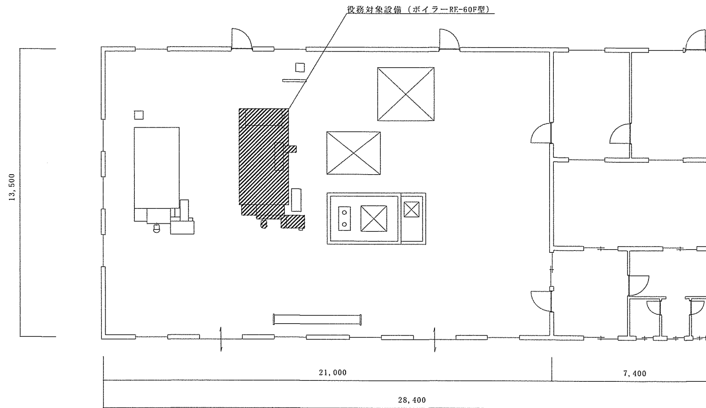
28号建物平面図 S=1:150
