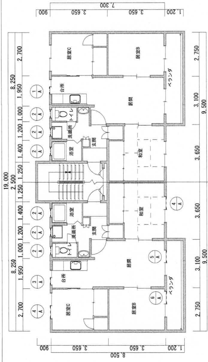
第2大津宿舍4号棟 標準平面図 S=1:150
