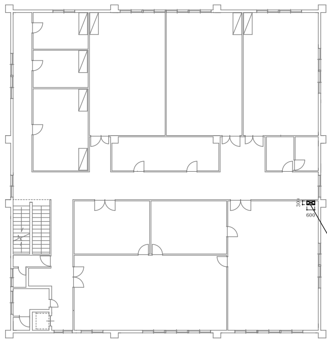
4 5 号建物平面図 S=1/300
