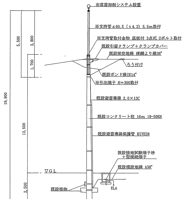
新設避雷針取付図 (基準) S=1/125
