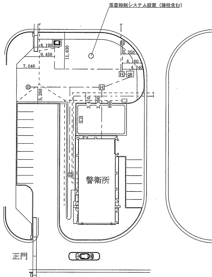
警衛所地域配置図 S=1/500
