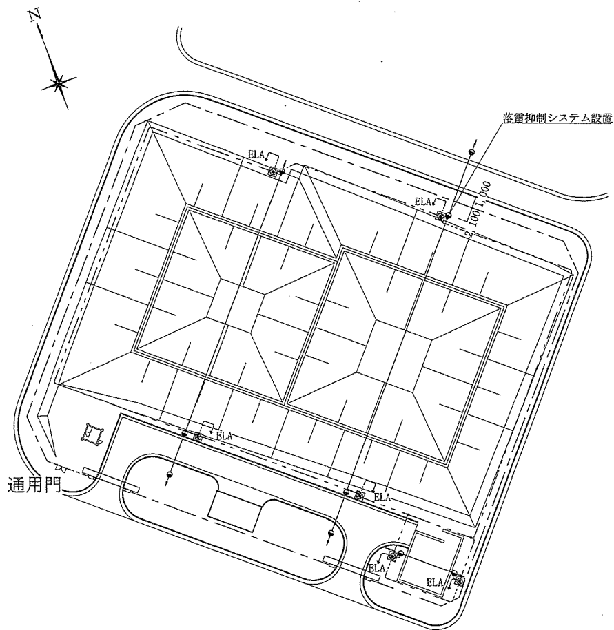
弾薬庫地域 配置図 S=1/750
