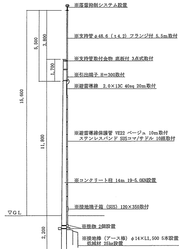
新設避雷針取付図 (基準) S=1/125
