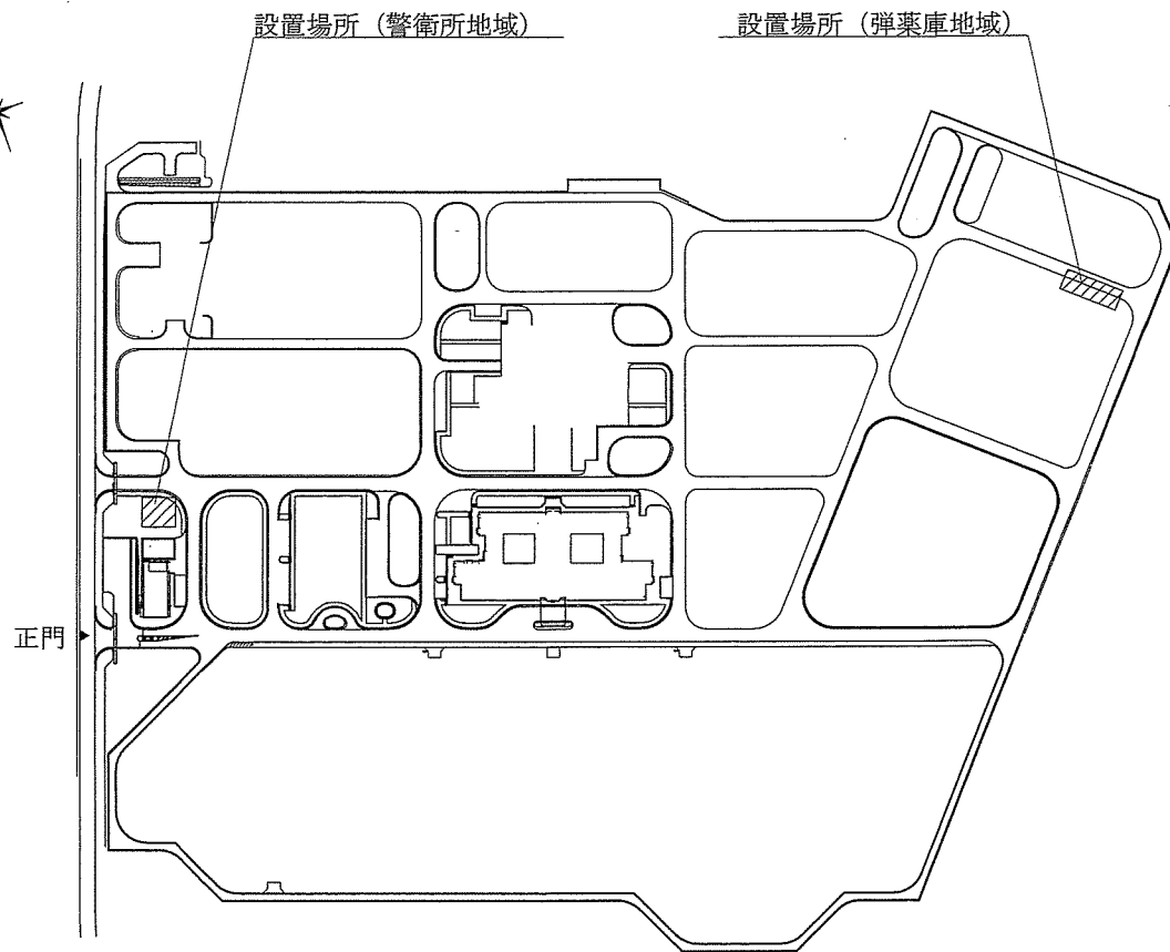
高知駐屯地配置図
