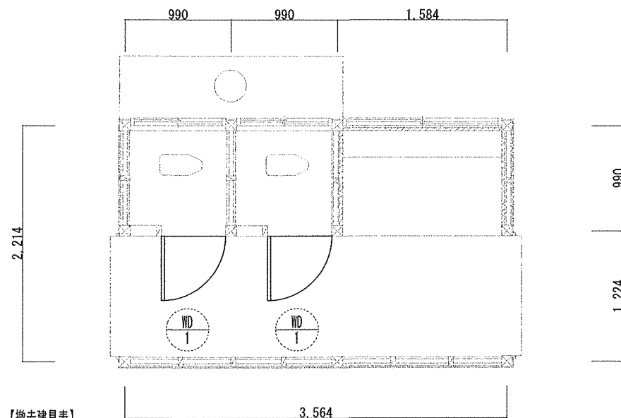
【撤去建具表】
