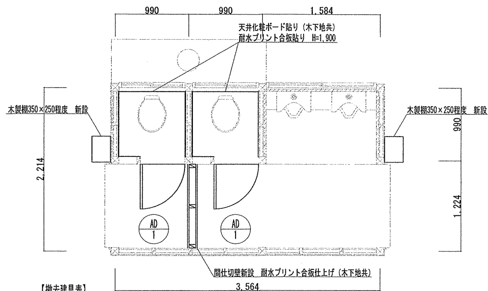
【撤去建具表】
