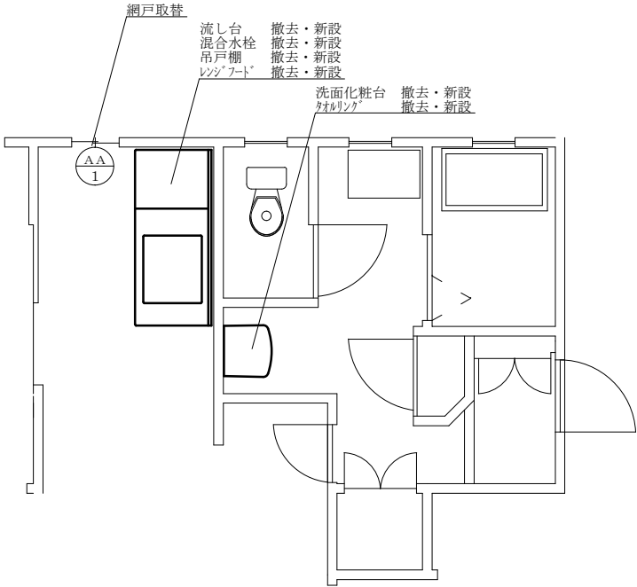
良蓮寺宿舎3号棟詳細平面図 S=1/50
