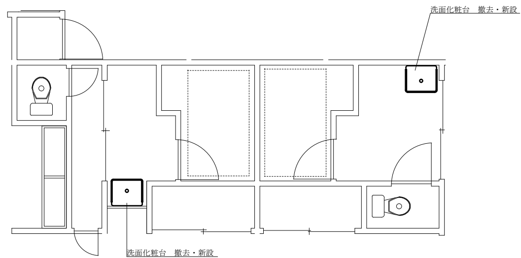
西宮宿舎詳細平面図 S=1/50
