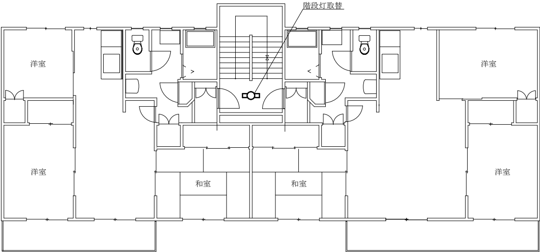
良蓮寺宿舎3号棟平面図 S=1/100
