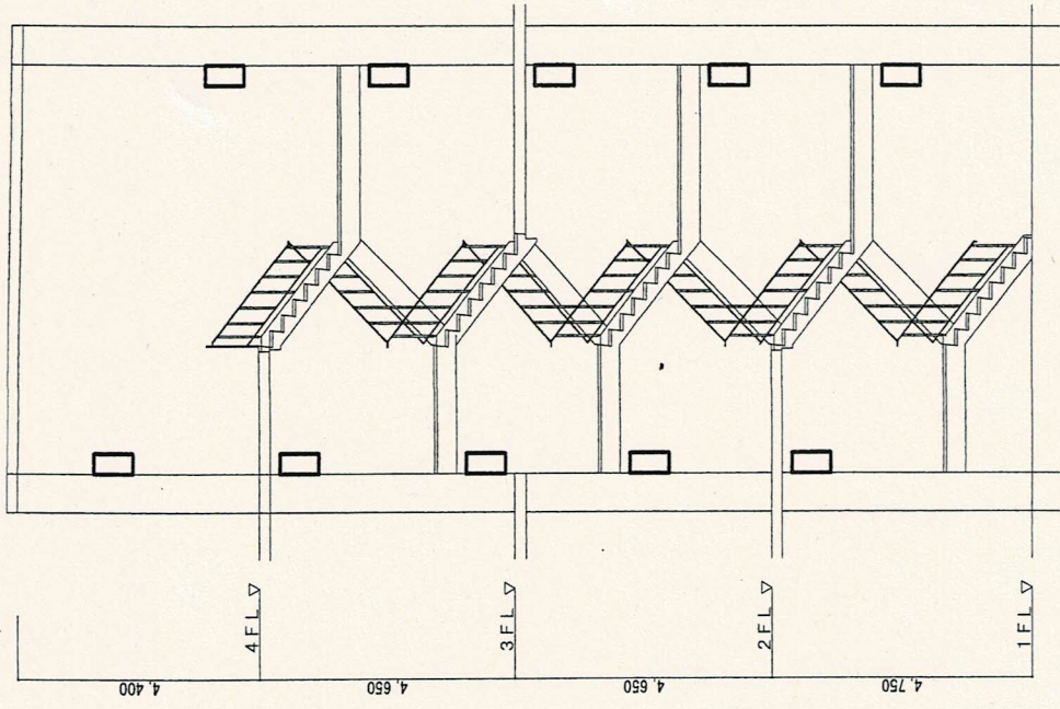
階段室断面図 1:150
