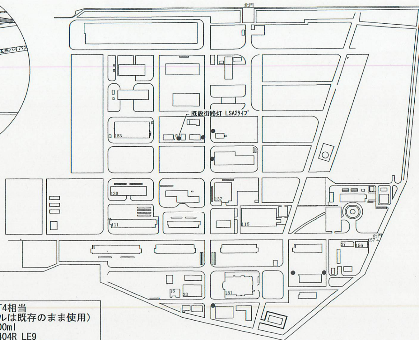
取替外灯配置図 S=1:4500
