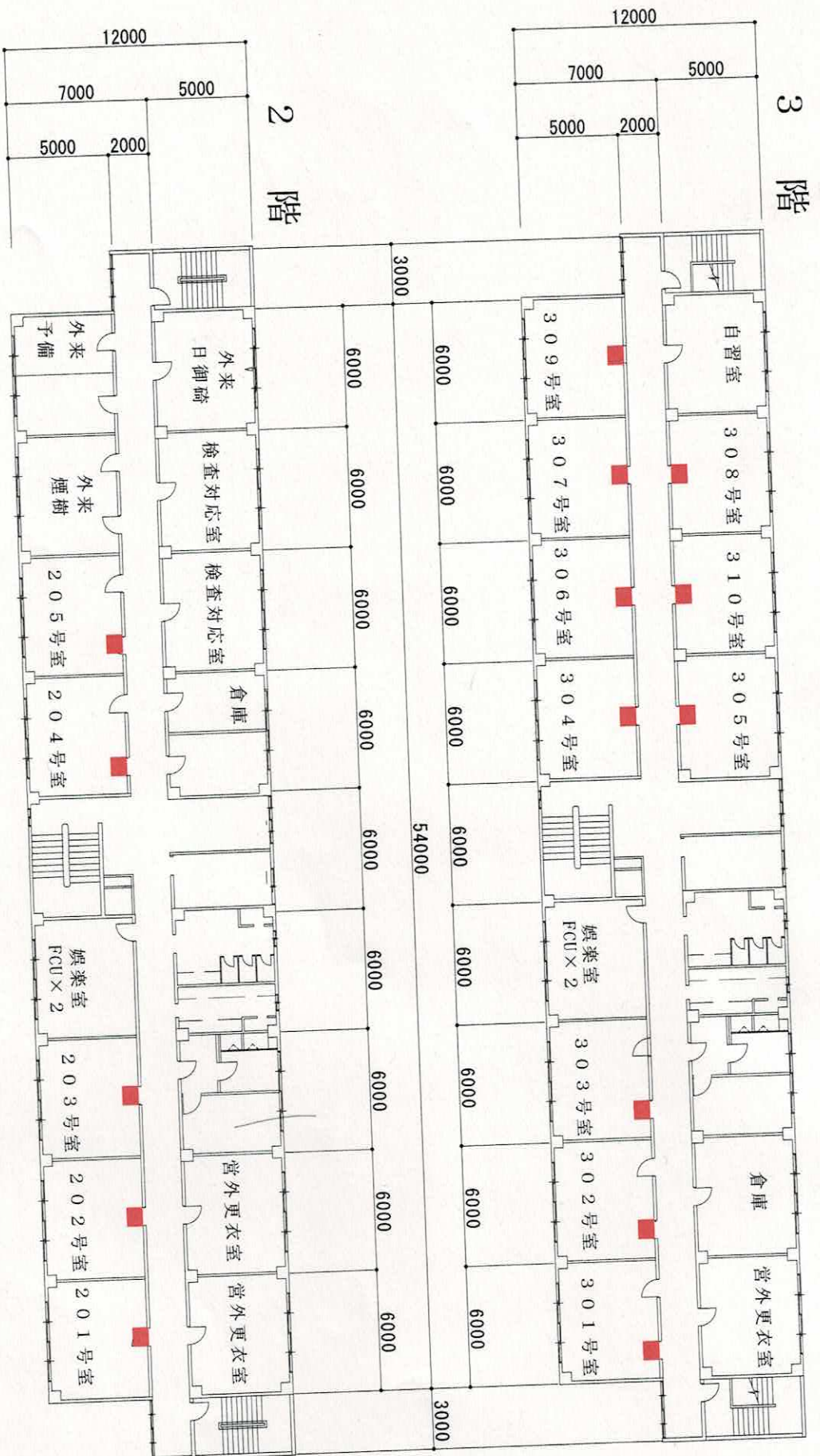
24号生活隊舎平面図
