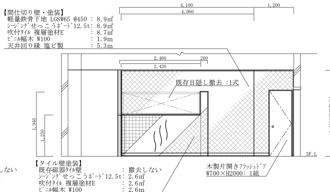
B面立面断面詳細図 S=1:50
