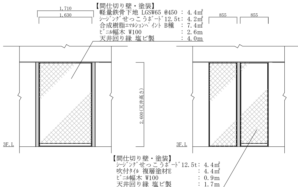
G-G' 立面断面詳細図 S=1:50
