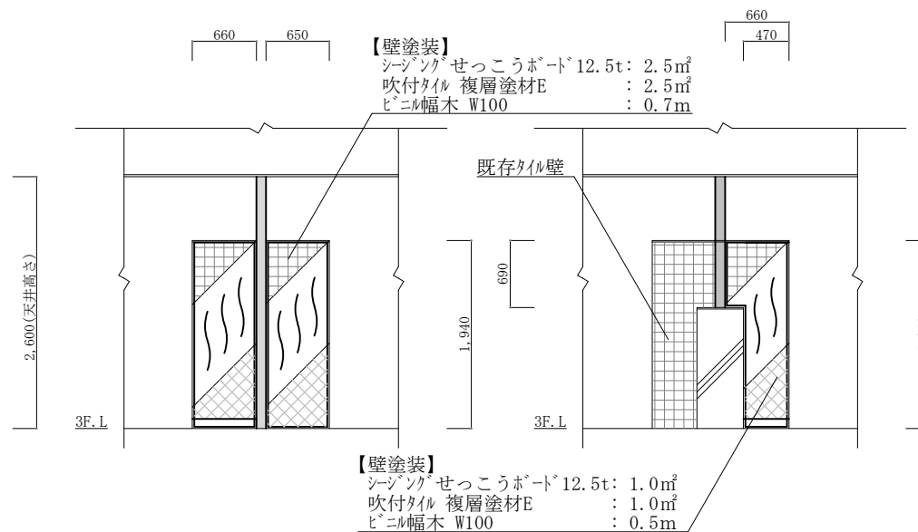
I-I' 立面断面詳細図 S=1:50
