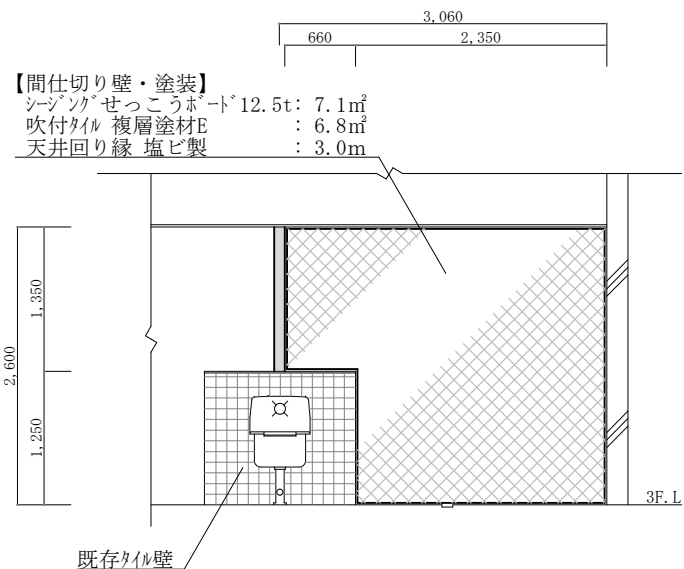
E-E' 立面断面詳細図 S=1:50
