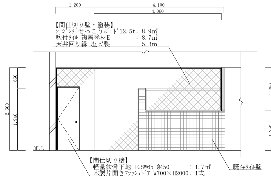
F-F' 立面断面詳細図 S=1:50
