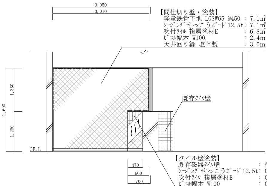
A面立面断面詳細図 S=1:50
