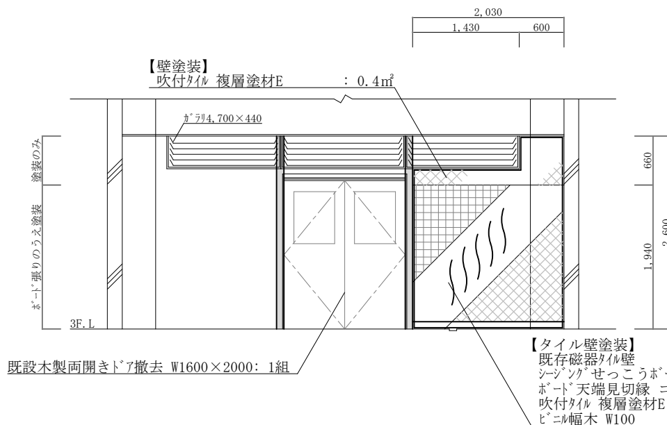
C面立面断面詳細図 S=1:50
