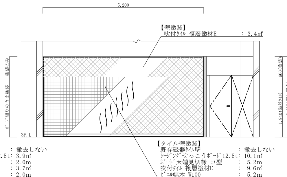
D面立面断面詳細図 S=1:50
