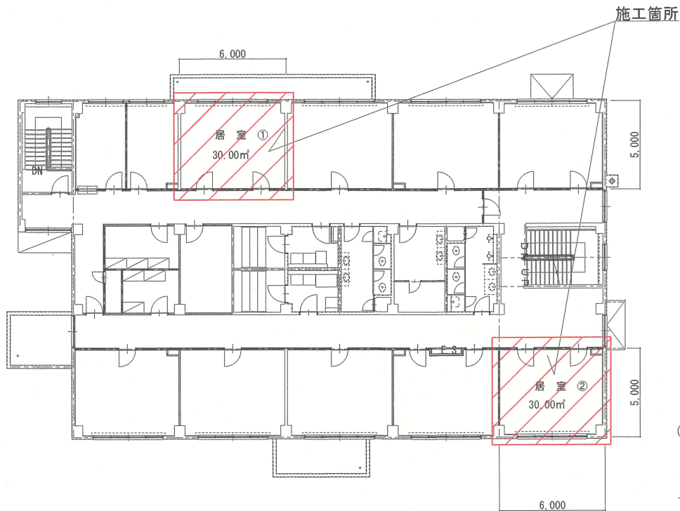
合棟隊舎 2階平面図
