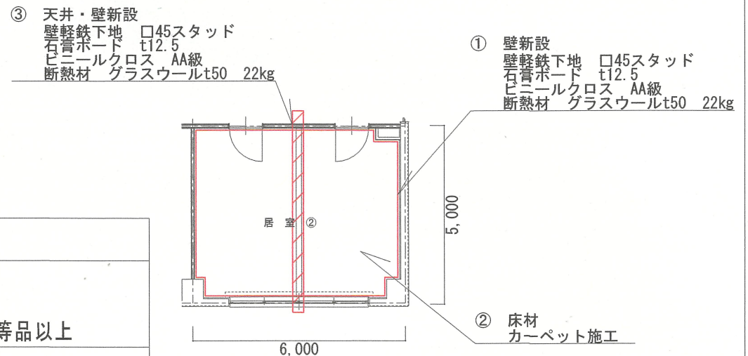
居室② 改修要領
