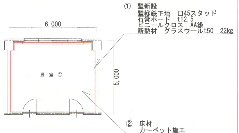
居室① 改修要領
