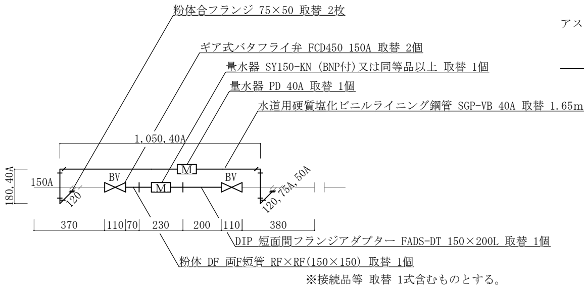
高架水槽付近量水器取替図 S=1/20
