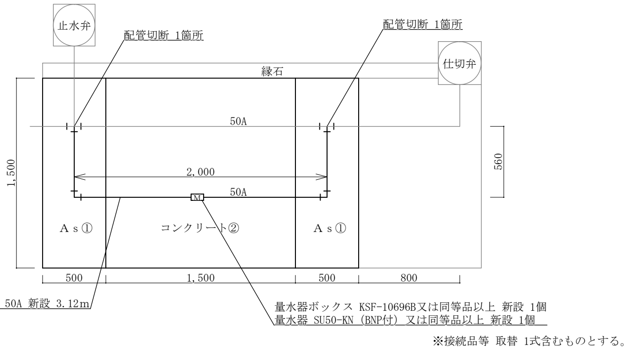
E 格納庫付近量水器新設図 S=1/20
