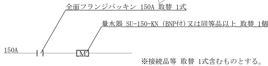
給水所付近量水器取替図 S=1/20
