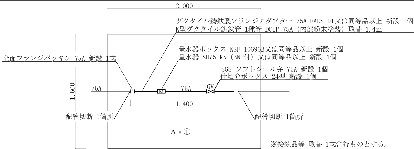
E 格納庫付近量水器新設図 S=1/20
