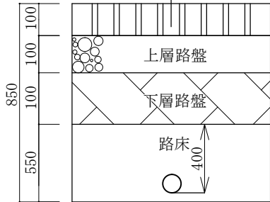
②断面図 S=1/NS
