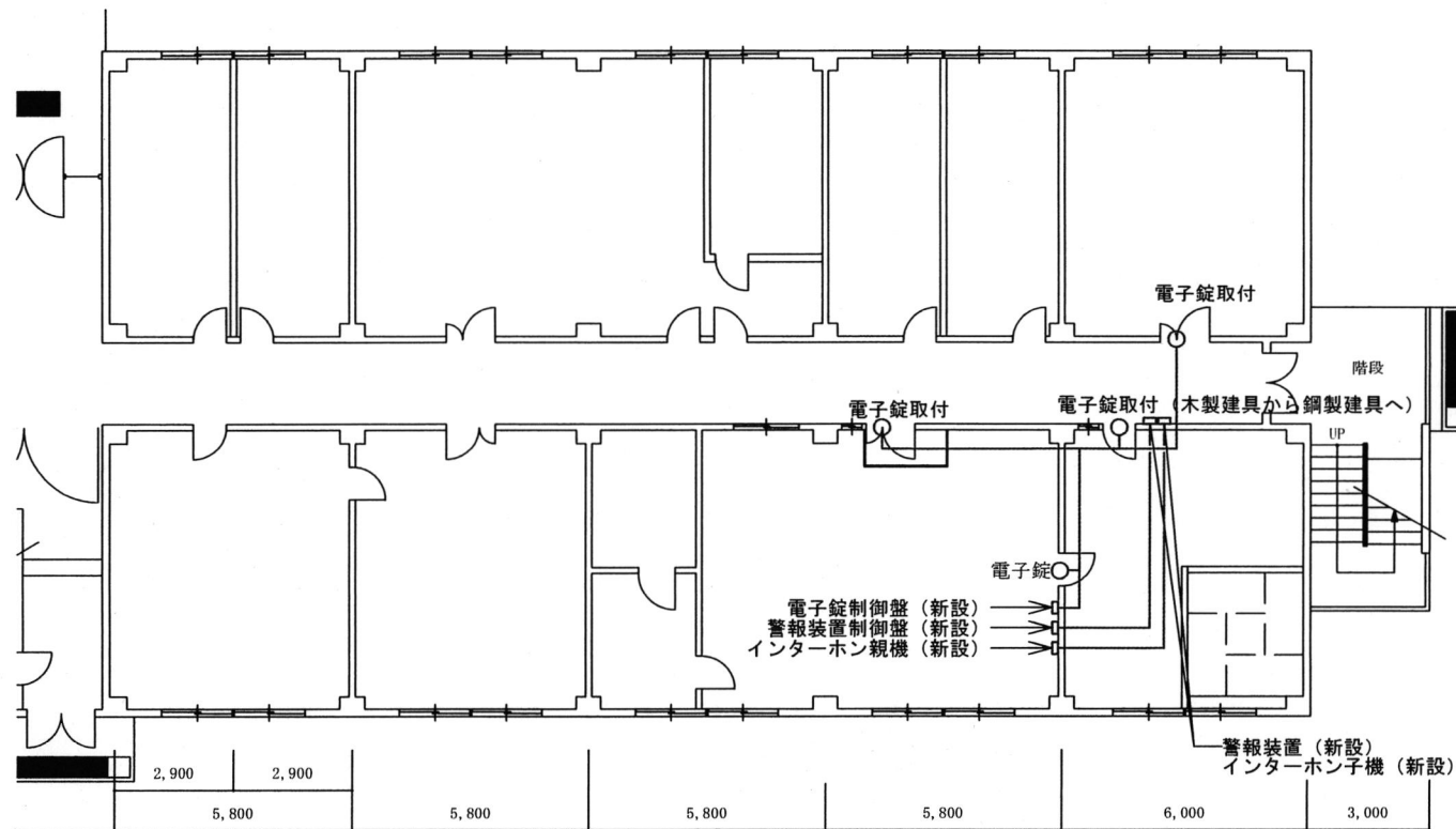
本部庁舎 1 階東側平面図 S=1:200
