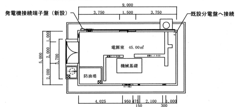
64号電源室平面図 S=1:200
