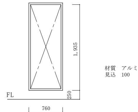
ユニットシャワー開口枠標準図
