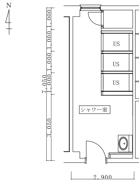
既設各階シャワー室平面図 S=1/100
