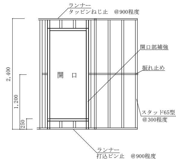
軽量鉄骨下地詳細標準図 S=1/50
