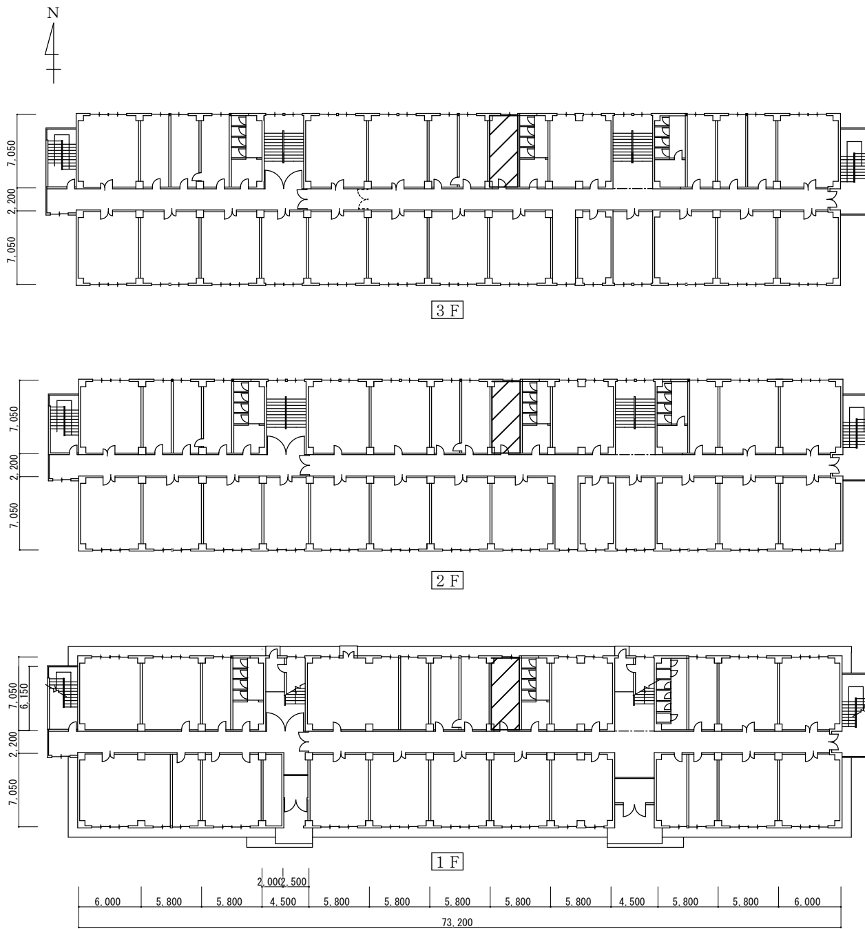
170号建物平面図 S=1/500
