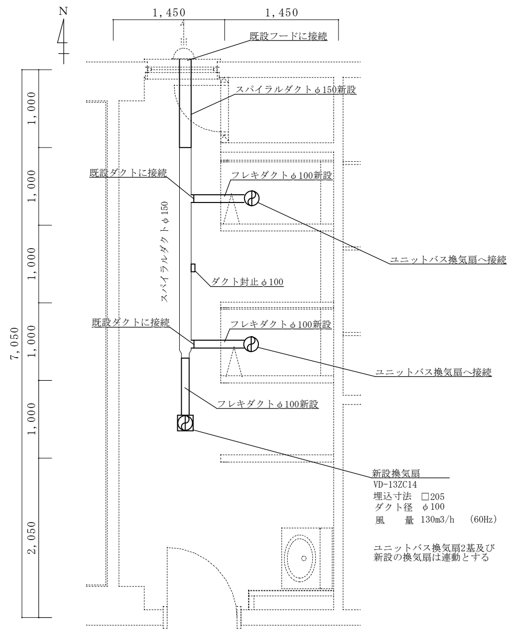
改修換気設備標準図 S=1/100
