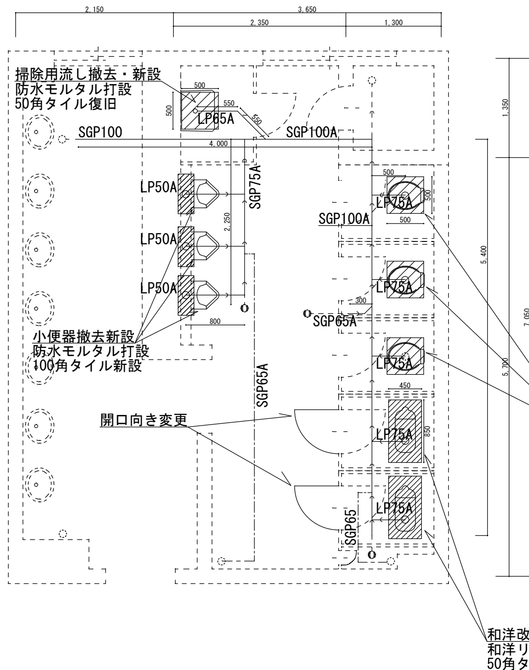
東側2～3階便所平面図（改修前） S=1/50
