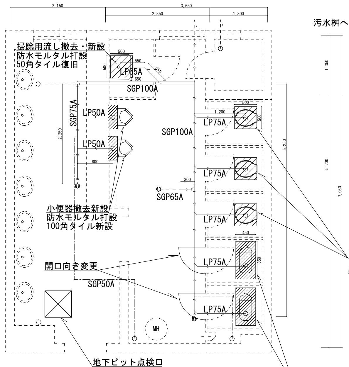
東側 1 階便所平面図（改修前） S=1/50
