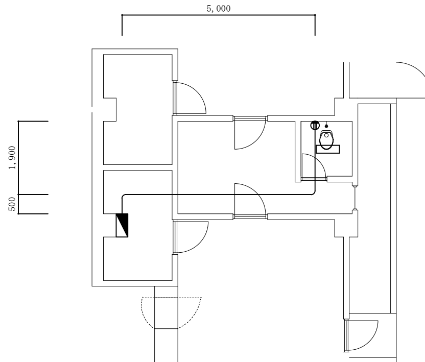
厚生センター 1 階③平面図 S = 1 : 1 0 0
