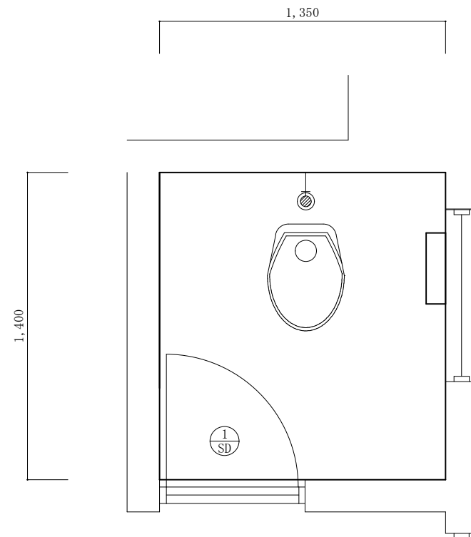
【改修後】厚生センター 1 階③便所平面図 S = 1 : 2 5
