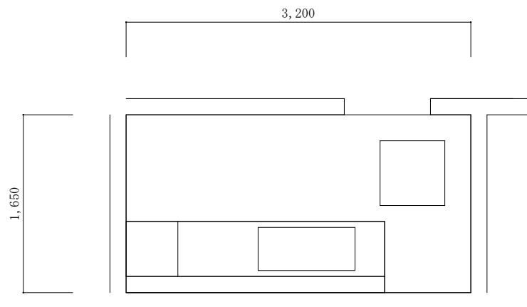
【改修前】厚生センター 1 階②便所平面図 S = 1 : 5 0
