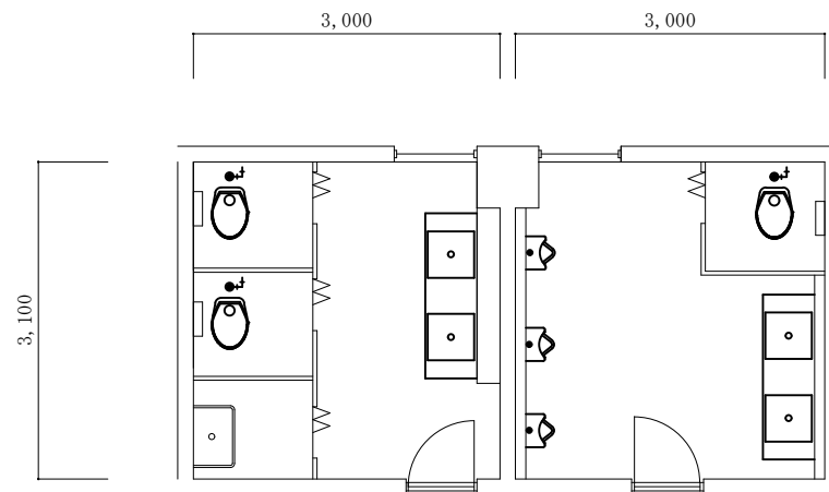
【改修後】厚生センター 2 階便所平面図 S = 1 : 8 0
