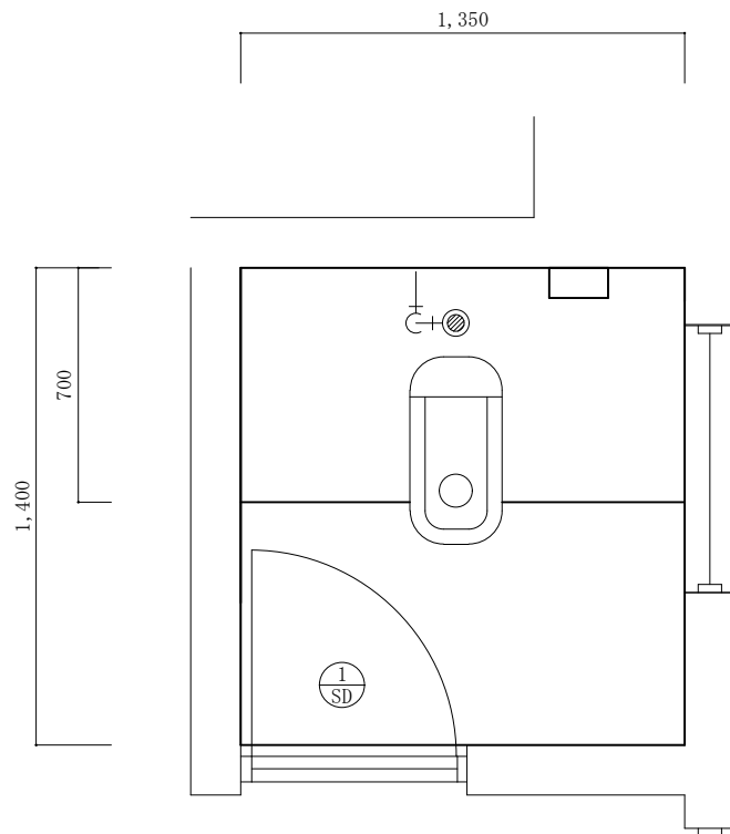
【改修前】厚生センター 1 階③便所平面図 S = 1 : 2 5
