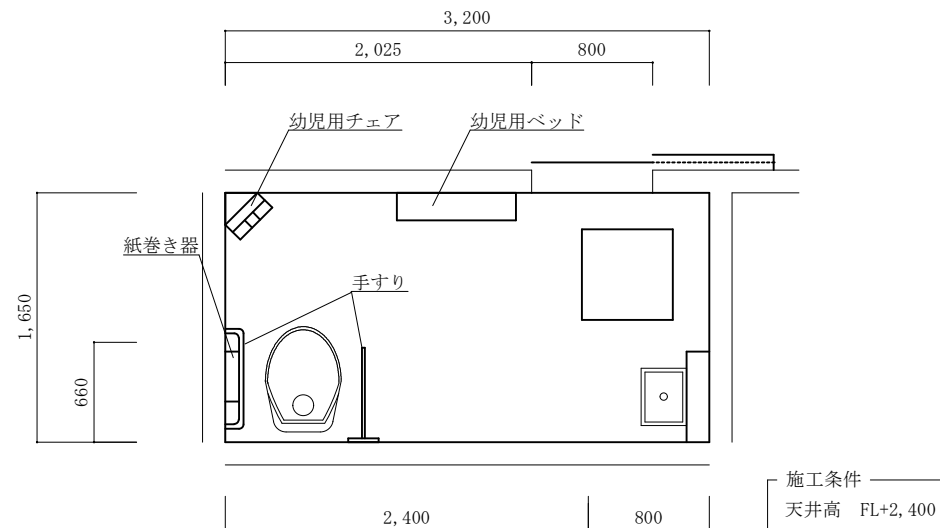
【改修後】厚生センター1階②便所平面図 S = 1 : 5 0
