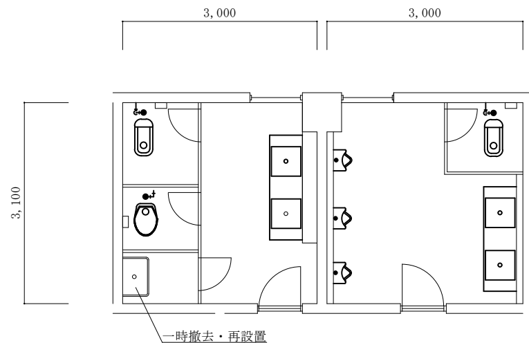
【改修前】厚生センター 2 階便所平面図 S = 1 : 8 0
