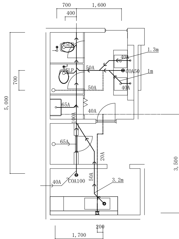
【改修前】厚生センター1階便所平面図 S = 1 : 1 0 0
