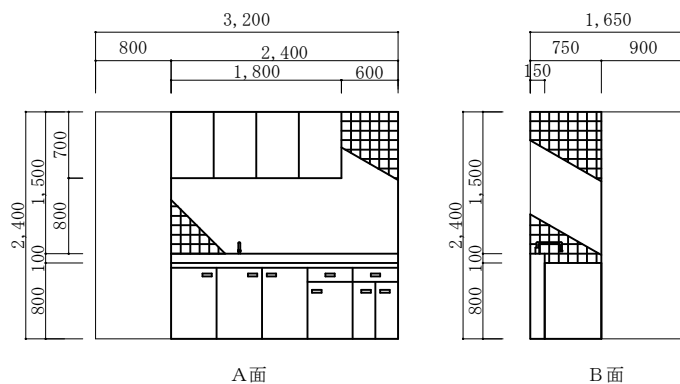
厚生センター1階②便所立面図 S = 1 : 8 0
