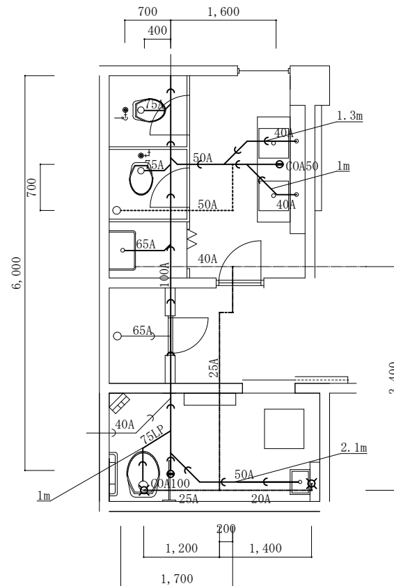
【改修後】厚生センター1階便所平面図 S = 1 : 1 0 0
