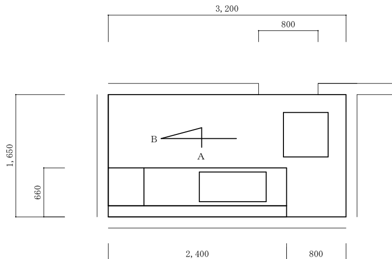
【改修前】厚生センター1階②便所平面図 S = 1 : 5 0
