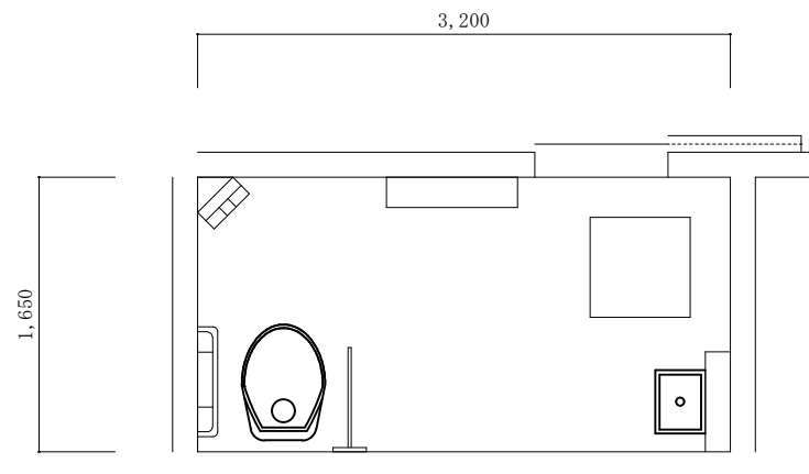
【改修後】厚生センター 1 階②便所平面図 S = 1 : 5 0
