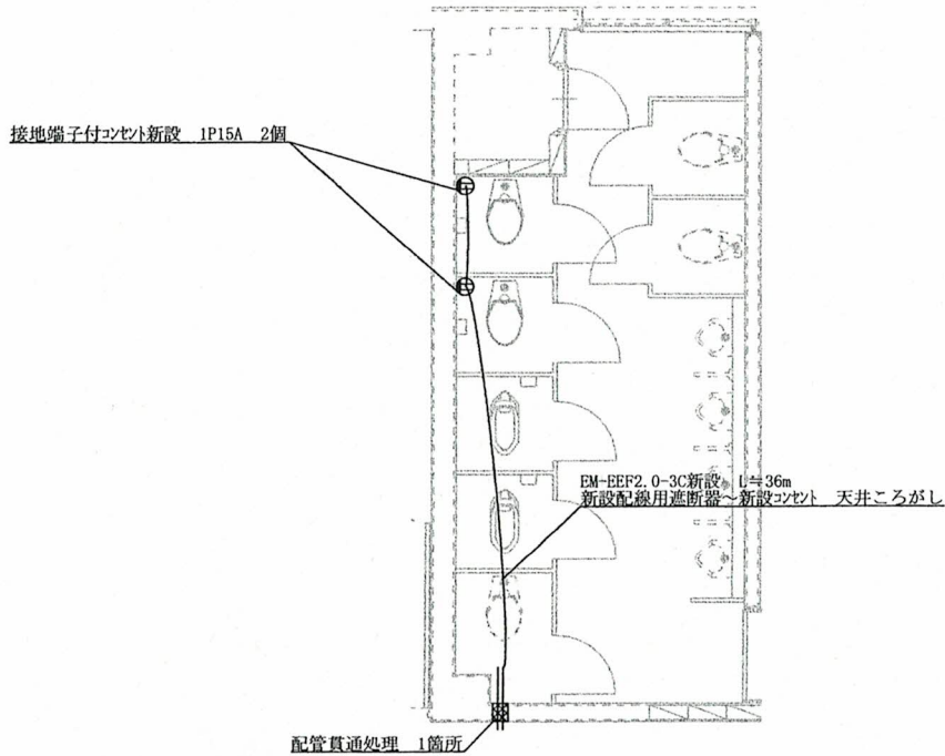
便所平面詳細図 (電気改修) S=1/文
