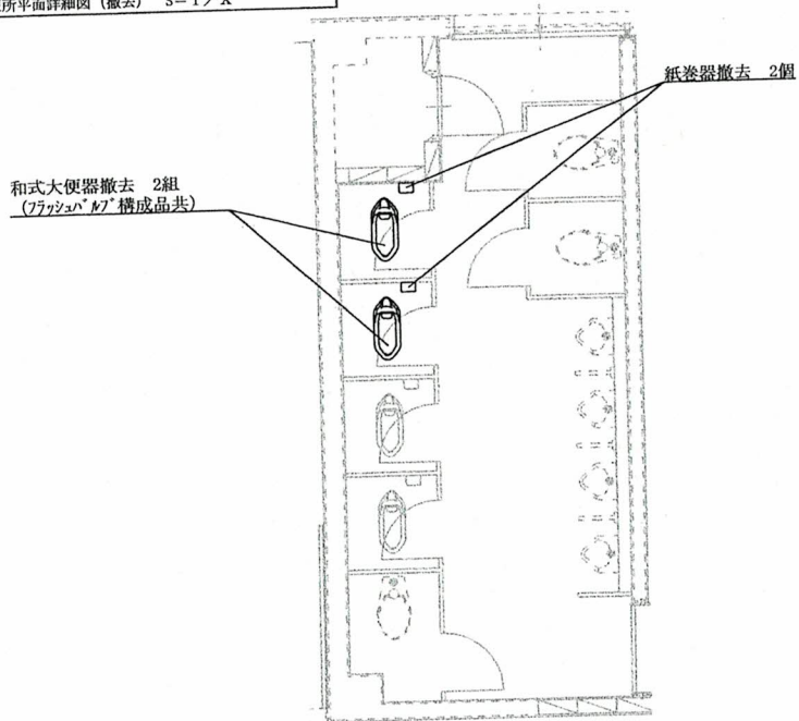
便所平面詳細図（撤去） S=1/X
