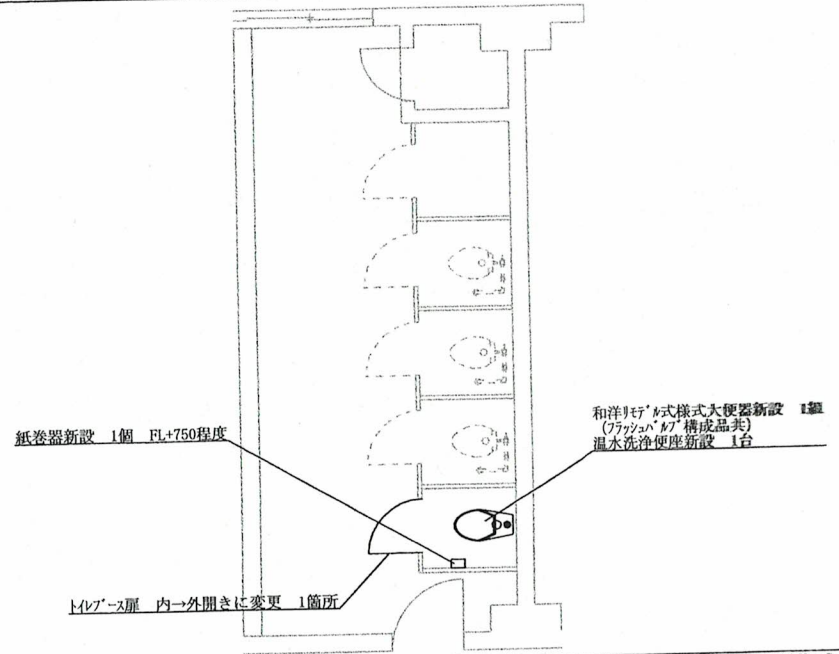
女子便所平面詳細図 (改修) S=1/X
