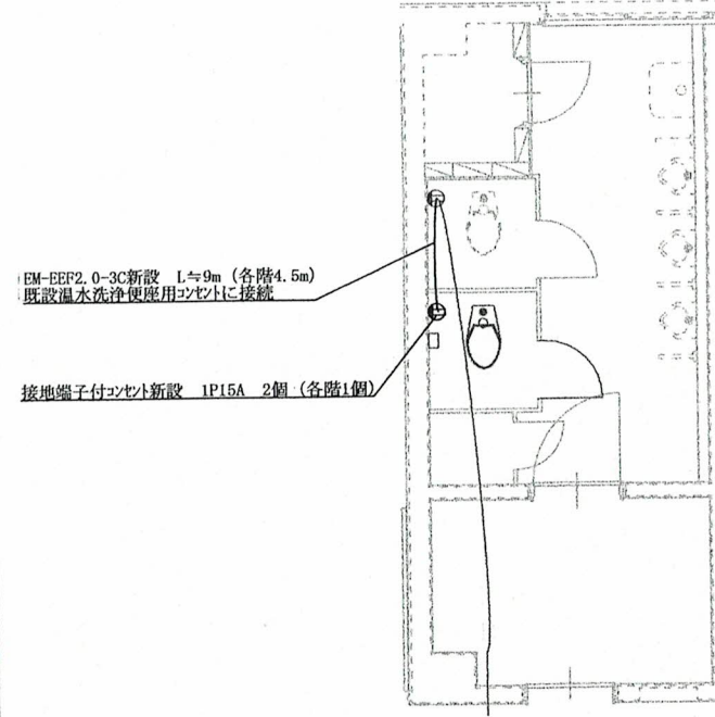
200号建物便所平面詳細図 (1~2階共通) (電気改修) S=1/X
