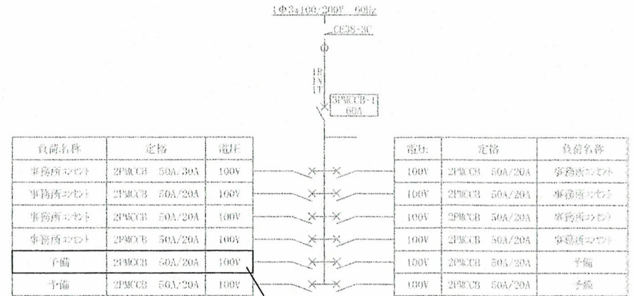
分電盤結線図 (電気改修) S=1/X
