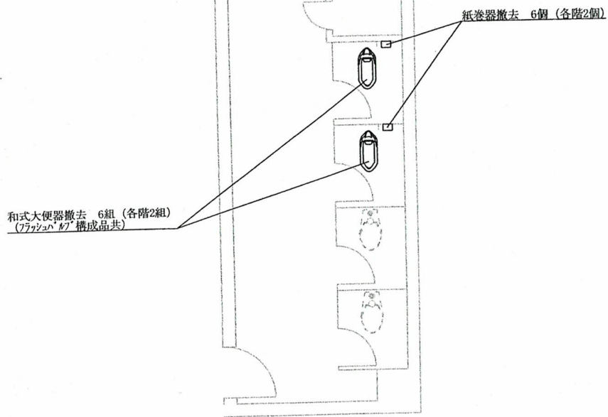
便所平面詳細図 (1~3階共通) (撤去) S=1/X
