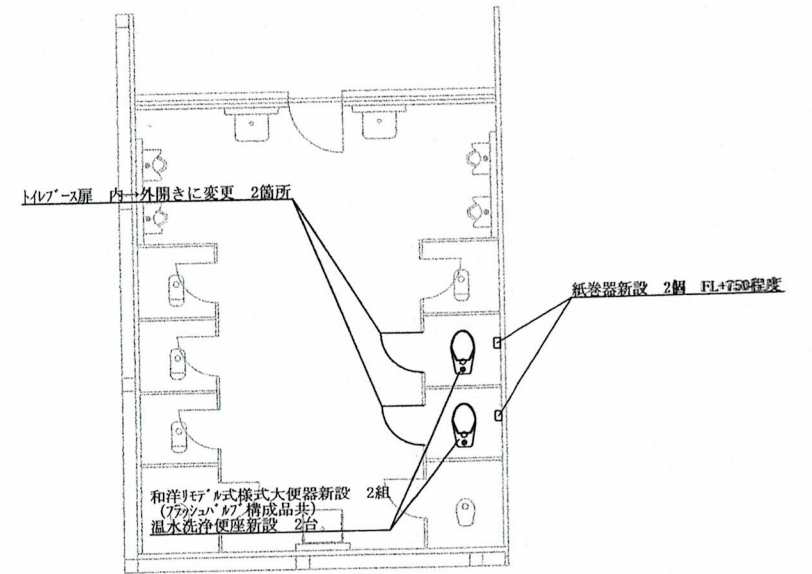
便所平面詳細図（改修） S=1/X
