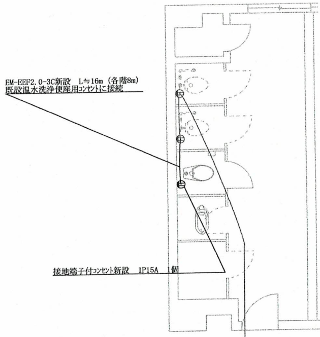
214号建物便所平面詳細図 (1~2階共通) (電気改修) S=1/X
