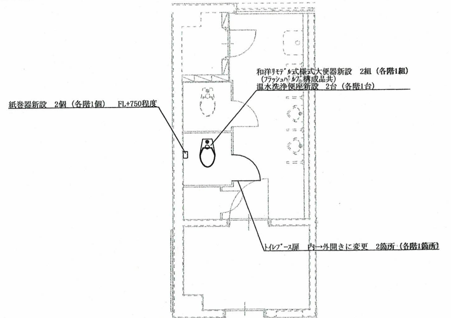
便所平面詳細図 (1~2階共通) (改修) S=1/X
