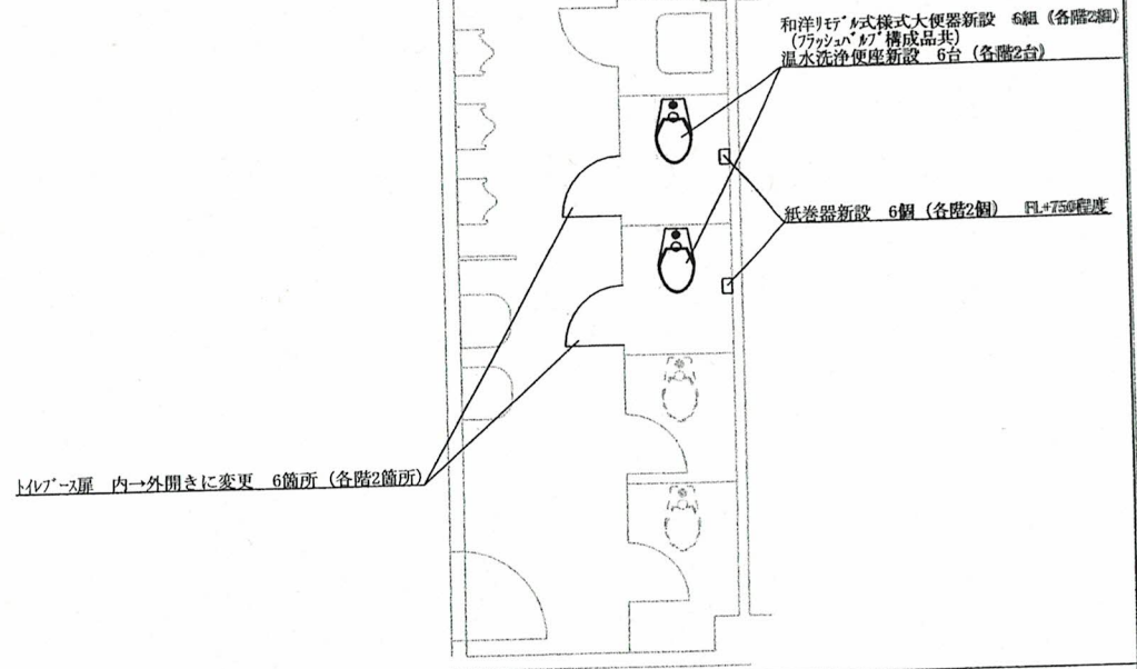
便所平面詳細図 (1~3階共通) (改修) S=1/X
