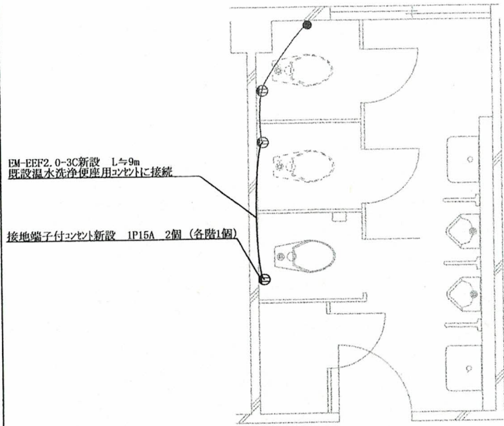
214号建物便所平面詳細図 (1~2階共通) (電気改修) S=1/X
