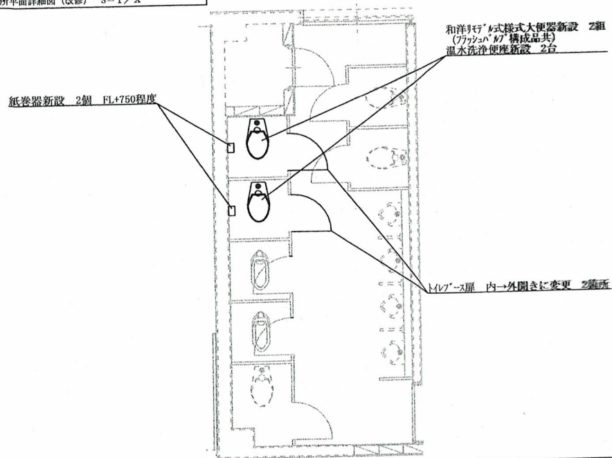
便所平面詳細図（改修） S=1/X
