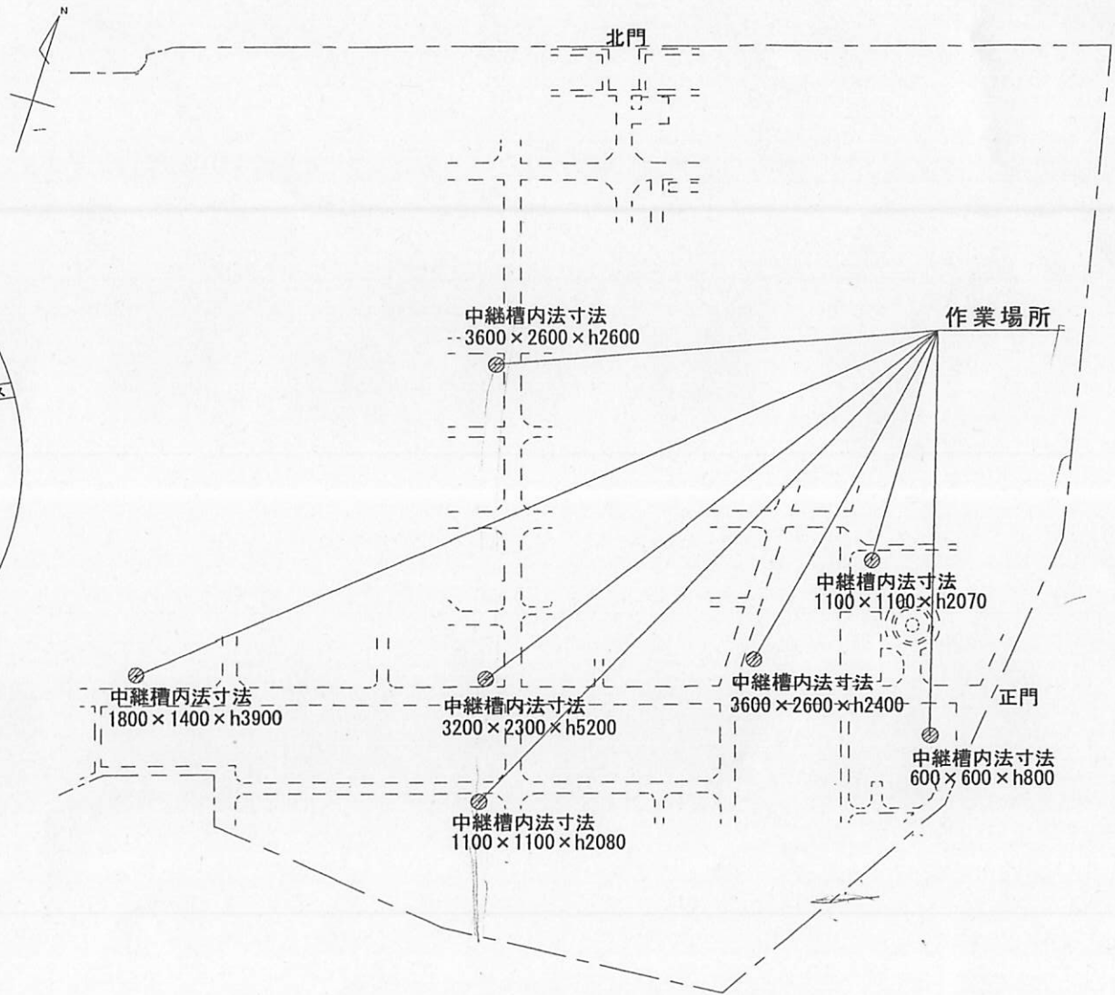
配置図 S=1:4500
