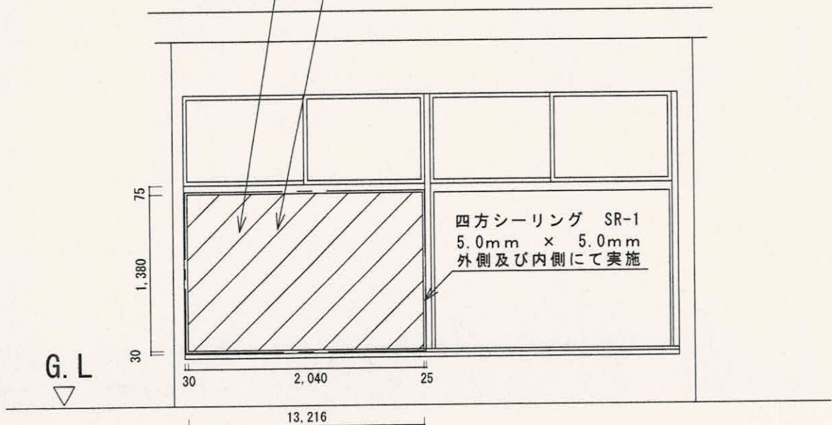
A-A' 詳細図 S=1:160
