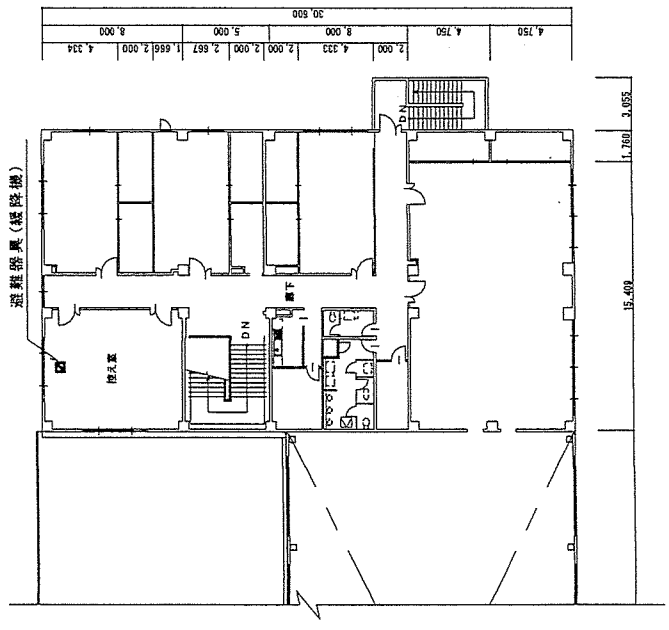
153号建物3階平面図
