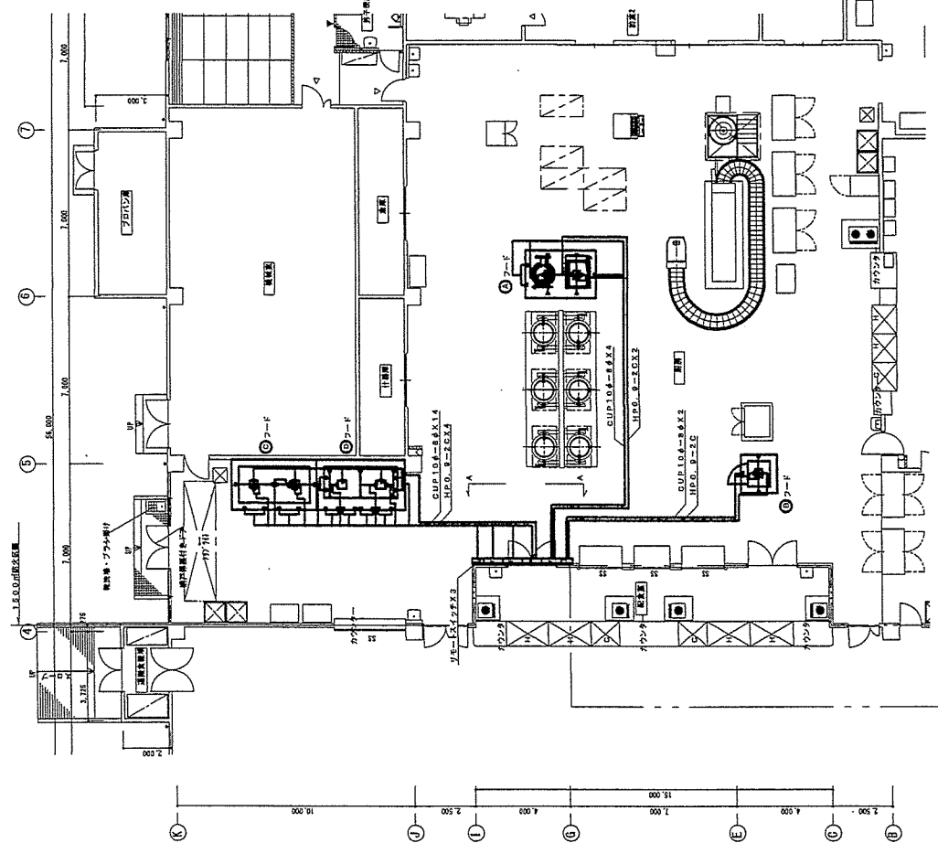
自動消火装置消防設備図
