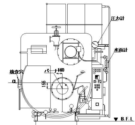
ボイラー正面詳細図
