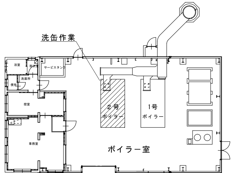
ボイラー室平面図 S = 1 : 300
