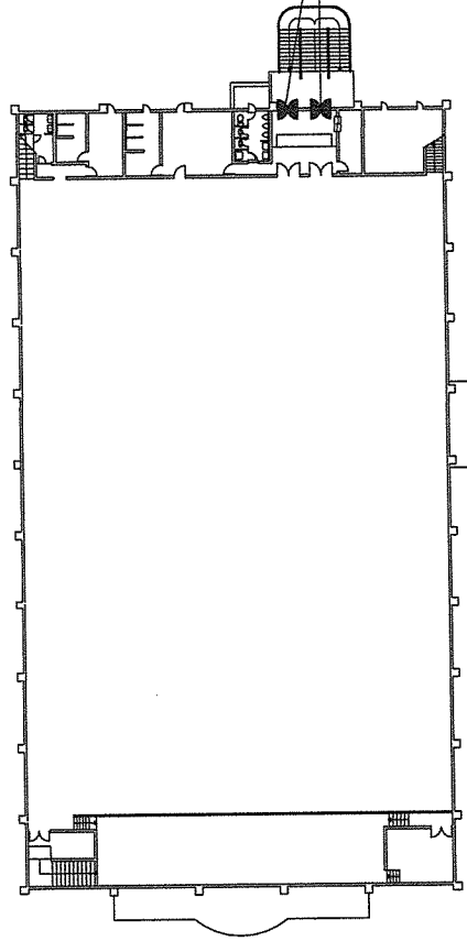
115号建物2階平面図 S=1/300
