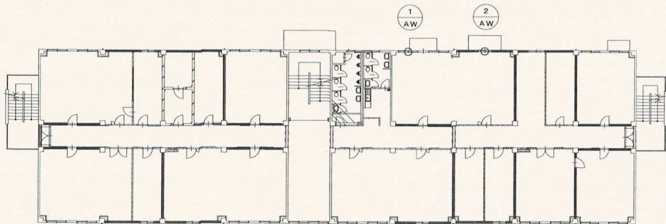
3号建物2階平面図 S = 1/X
