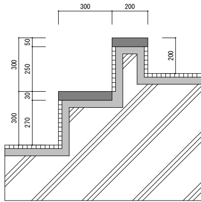
S = 1 / 1 5 A - A ' 断面図
