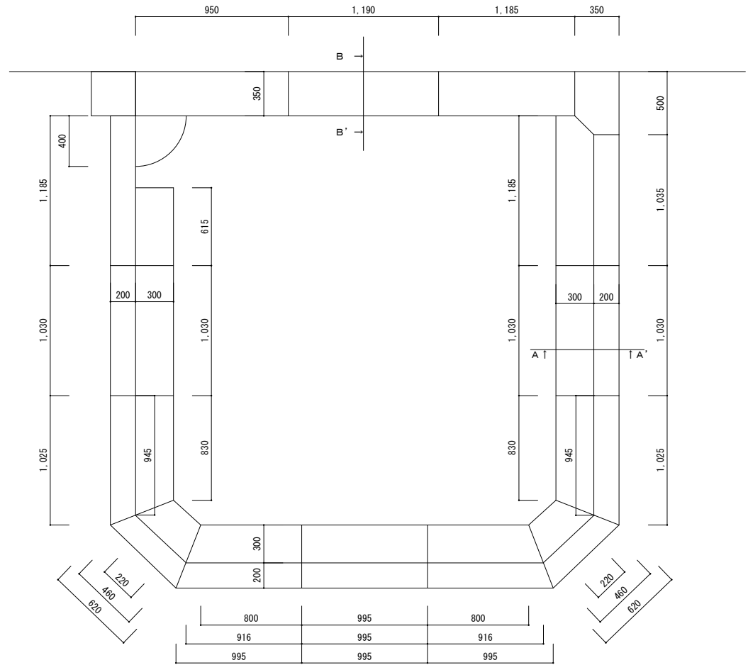
S = 1 / 3 0 浴槽平面図
