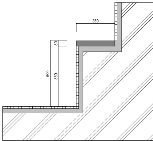
S = 1 / 1 5 B - B ' 断面図
