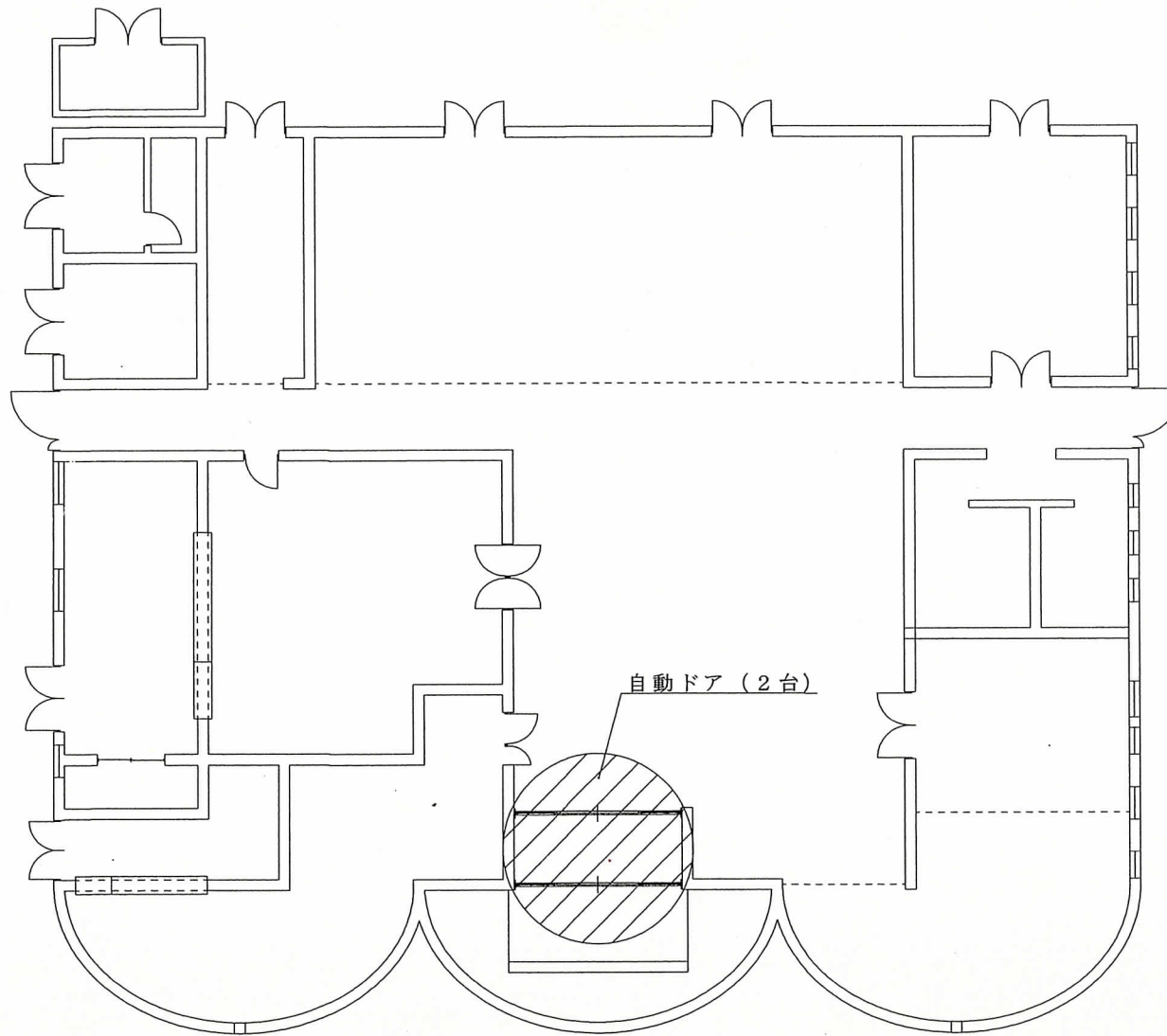
87号厚生センター平面図 S=1:200
