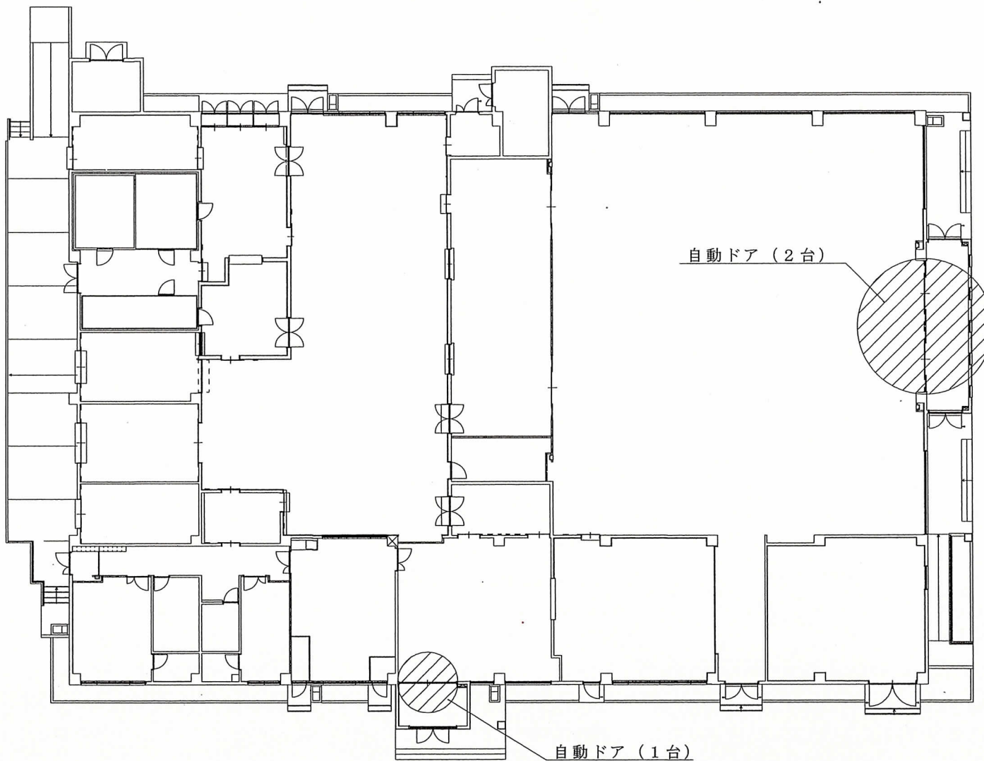
89号食厨平面図 S = 1 : 300
